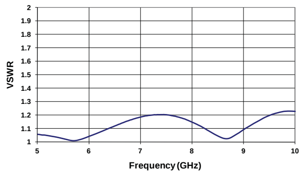
VSWR (5-10 GHz)
