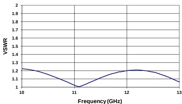
VSWR (10-13 GHz)
