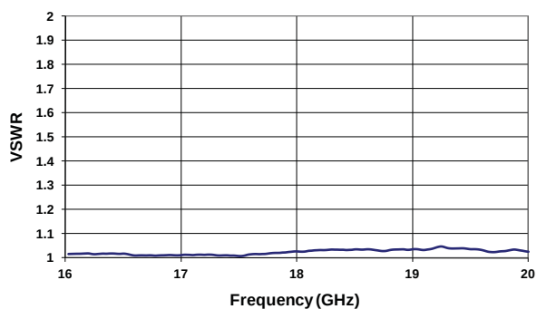
VSWR ( 16-20 GHz )
