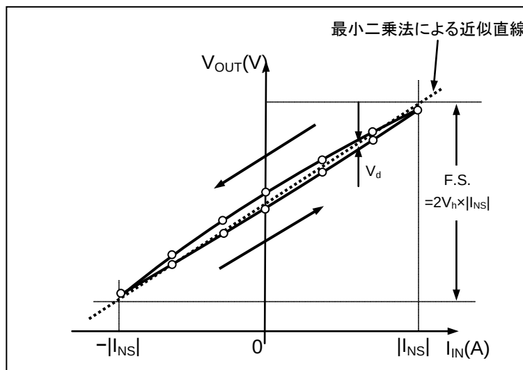
Figure 5. CQ-2233の出力特性
