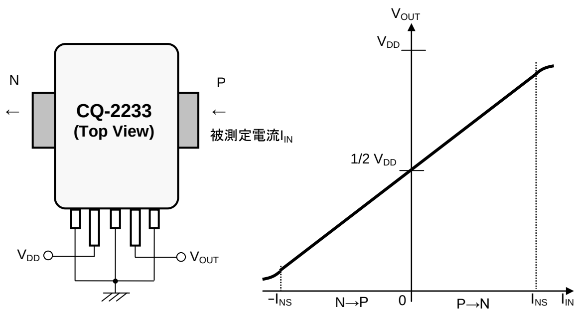
Figure 2. CQ-2233の出力特性
