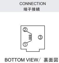
BOTTOM VIEW/ 裏面図
