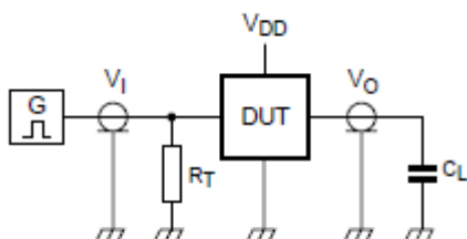
图 9 测试电路
