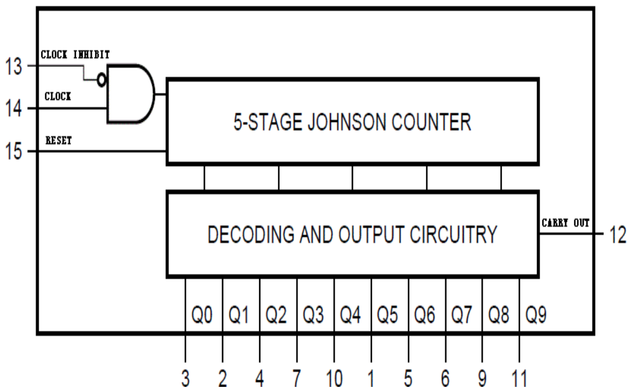
图 1 功能框图
