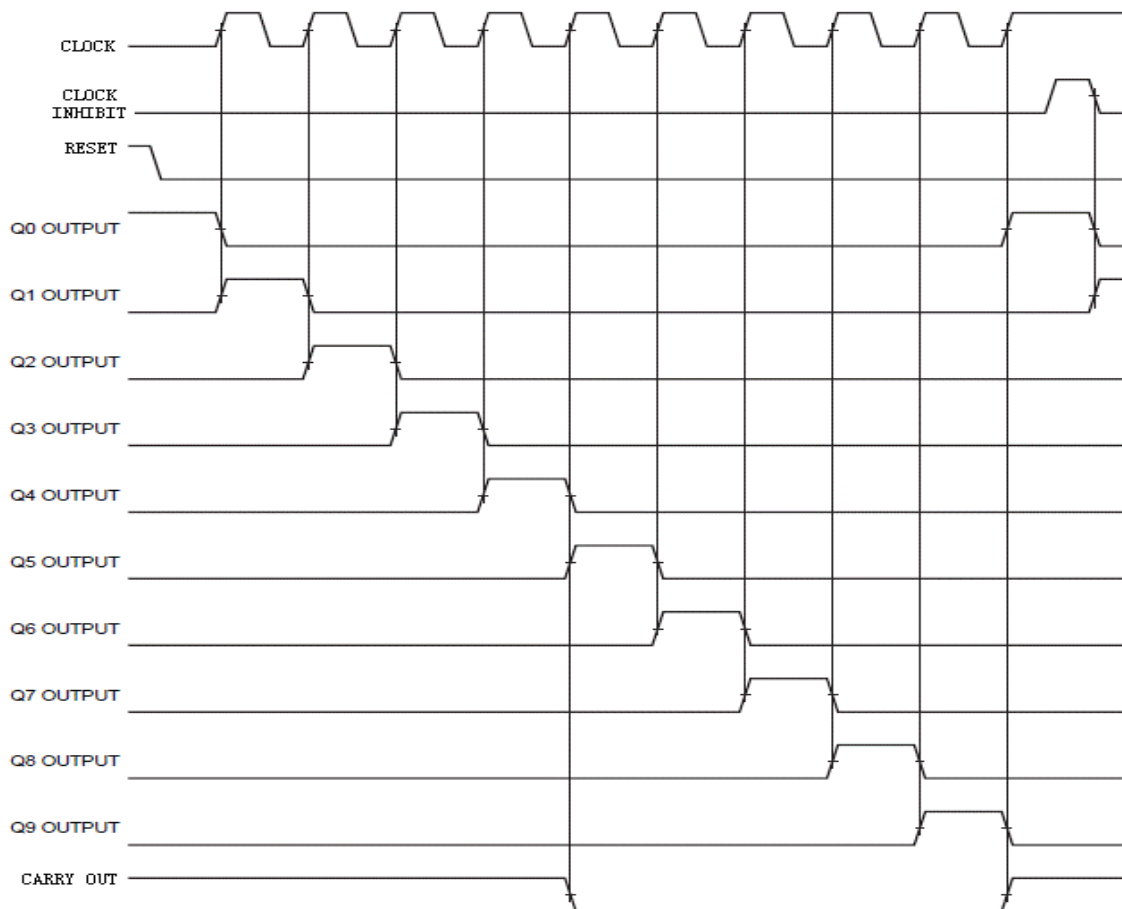
图 5 时序图
