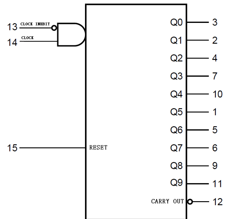
图 2 逻辑符号
