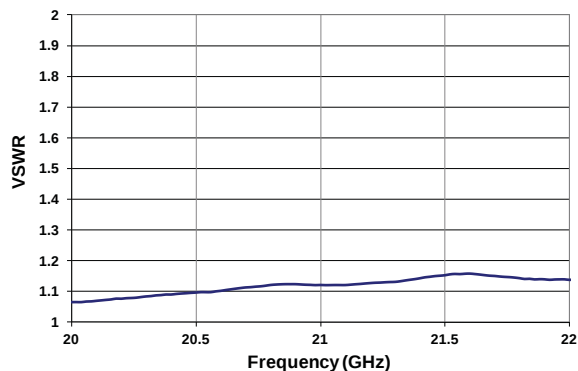
VSWR ( 20-22 GHz )
