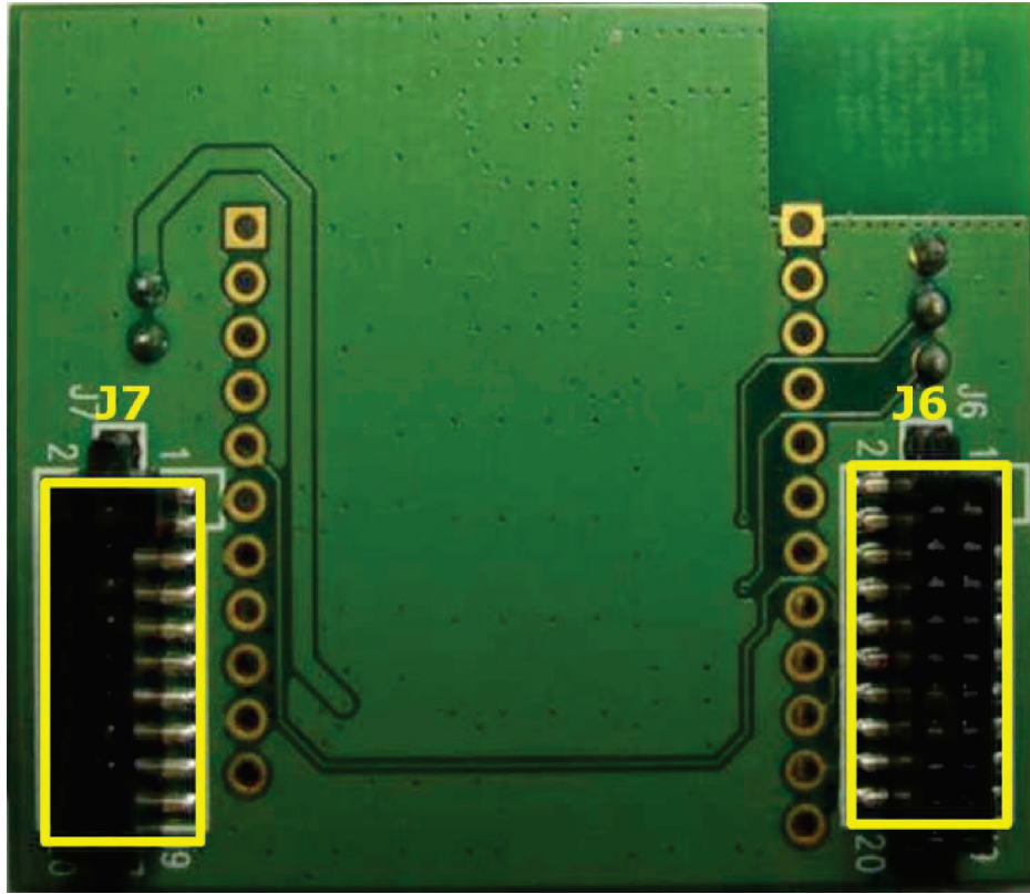
Figure 2-2. CC3000 EM Board Bottom View
