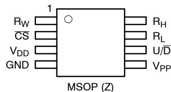
MSOP (Z)
