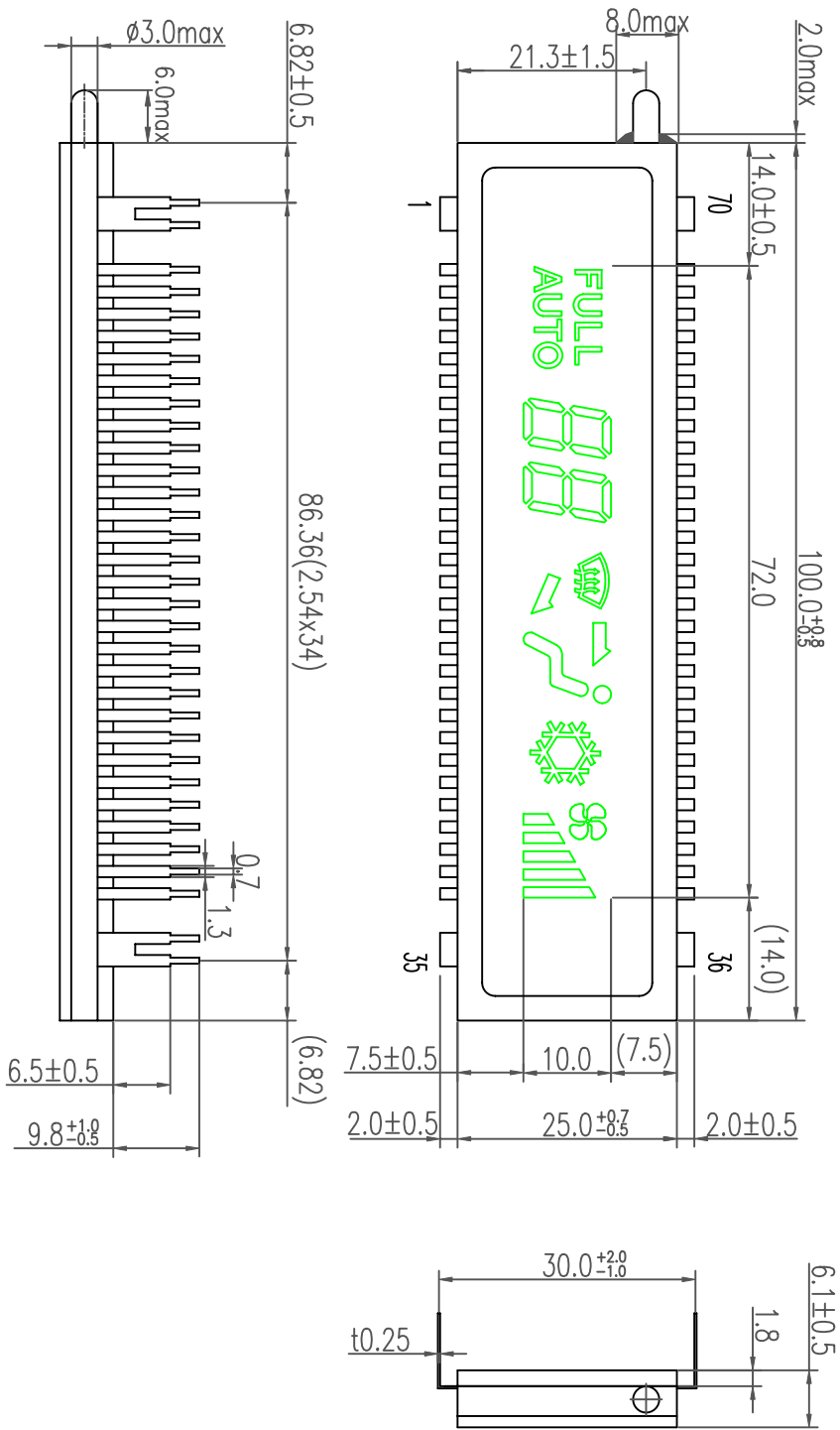
管脚连接 (PIN CONNECTION)
