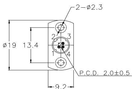
FC Receptacle
