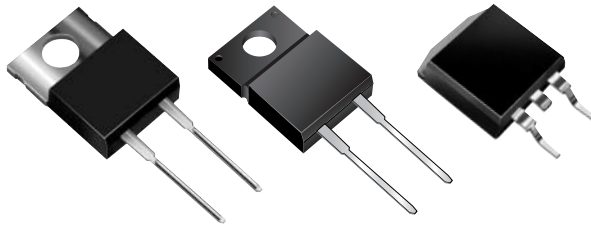
TO-220AC (BYS459)
