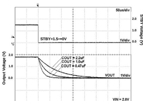
Fig 26. Discharge Time
