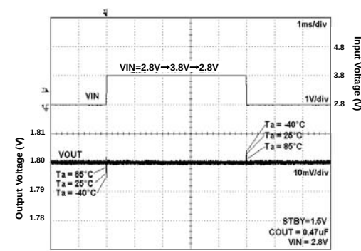
Fig 27. VIN Response
