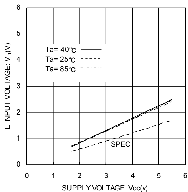
Fig.5 'L' input voltage V_{IL1} (A0,A1,A2,SCL,SDA,WP)
