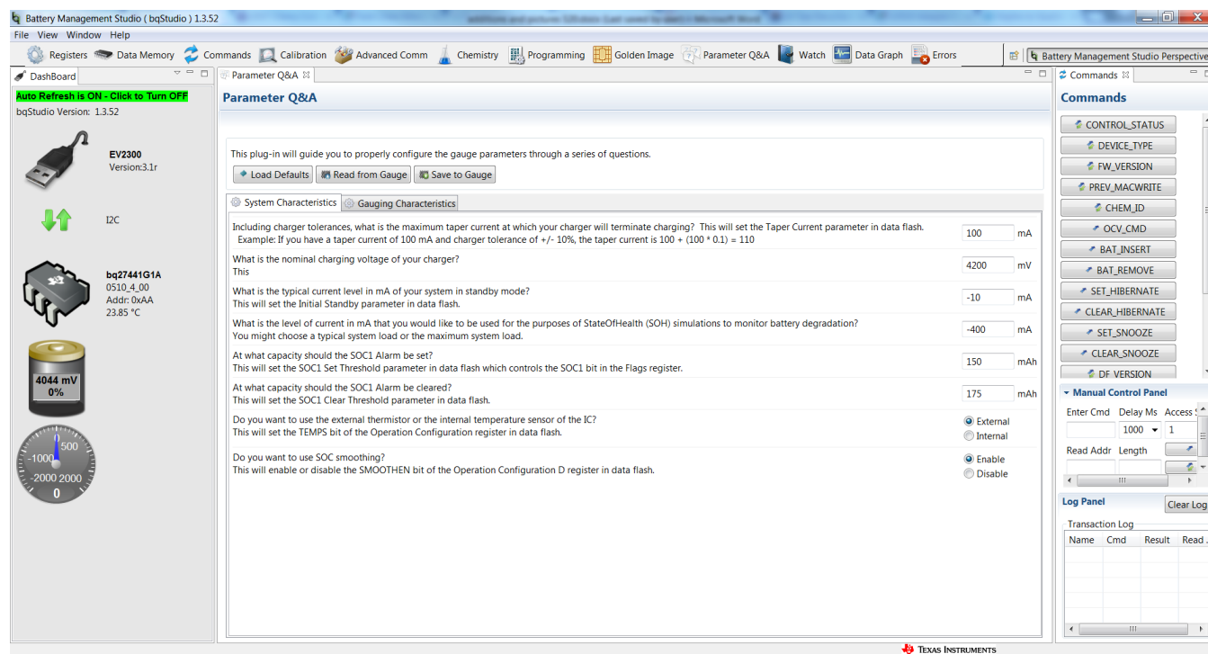
Figure 13. Parameter Q&amp;A Screen
