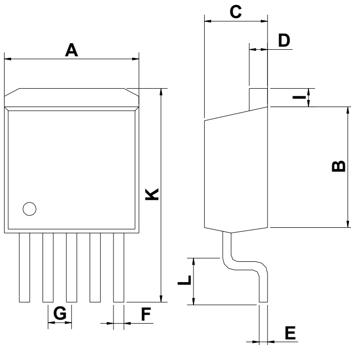
TO-263 (N263)
