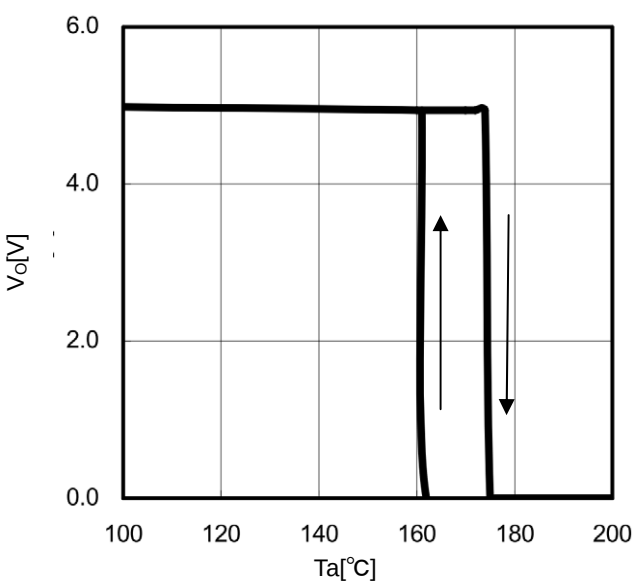
Figure 28. TSD (I o =0mA)
