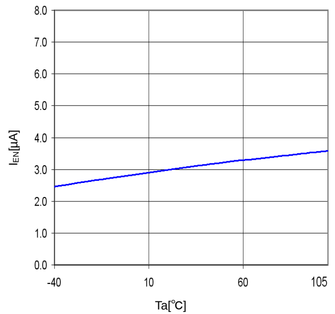
Figure 24. T a -I EN
