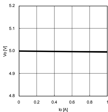
Fig.11 I_o - V_o
