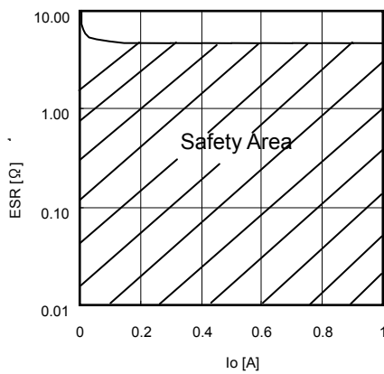
Fig.17 ESR condenser
