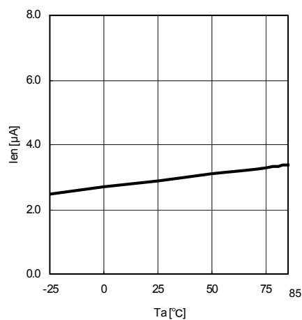
Fig.10 T_a - I_{EN}
