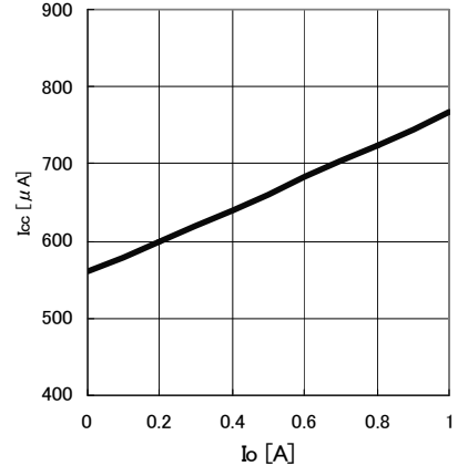
Fig.18 I_o-I_{cc}
