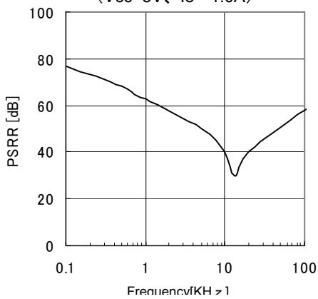
Fig.19 PSRR( I_o=0\text{mA} )
