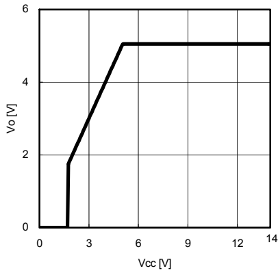
Fig.13 V_{cc}-V_o ( I_o=0\text{mA} )
