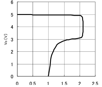
Fig.15 OCP
