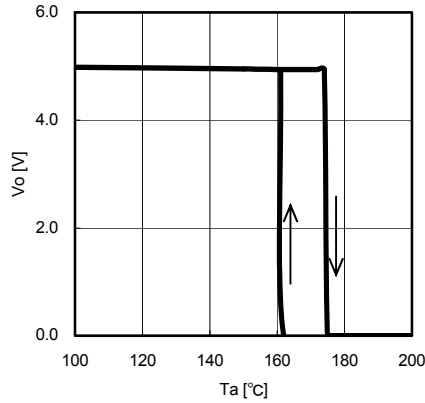
Fig.14 TSD ( I_o=0\text{mA} )
