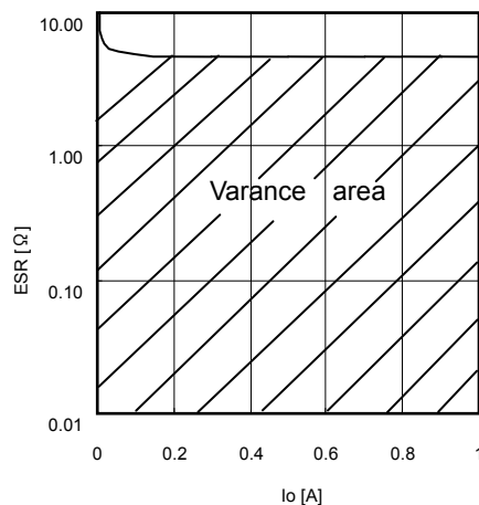
Fig.17 ESR condenser
