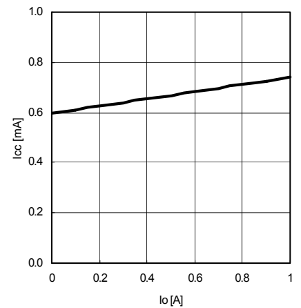
Fig.18 I_o - I_{cc}
