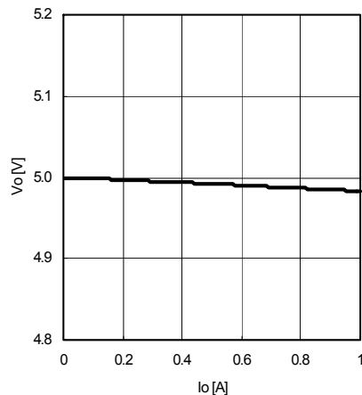
Fig.11 I_o - V_o
