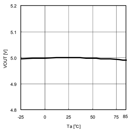
Fig.7 T_a - V_o ( I_o=0\text{mA} )
