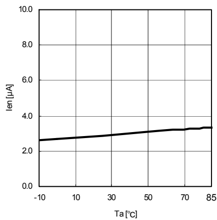
Fig.10 T_a - I_{EN}
