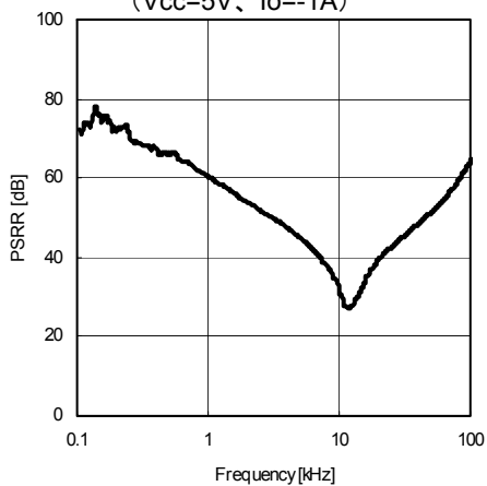
Fig.19 PSRR( I_o=0 mA)
