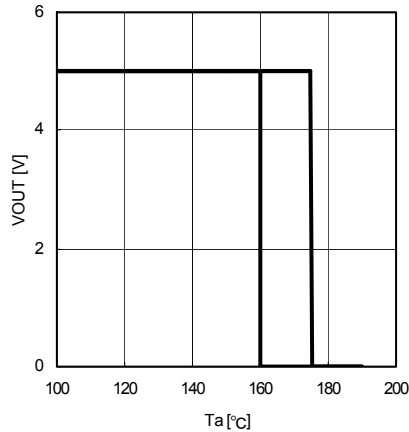
Fig.14 TSD ( I_o=0 mA)
