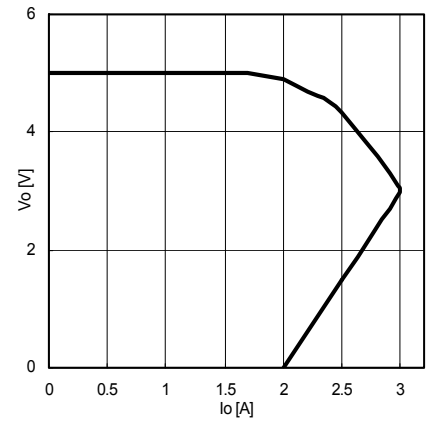
Fig.15 OCP
