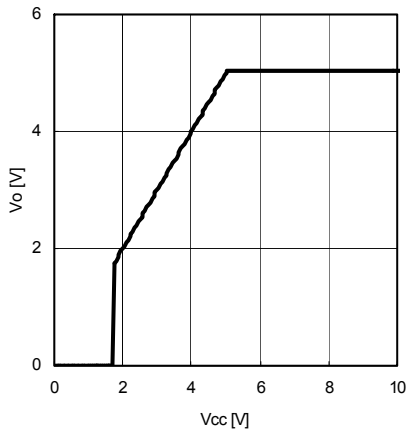
Fig.13 V_{cc} - V_o ( I_o=0 mA)
