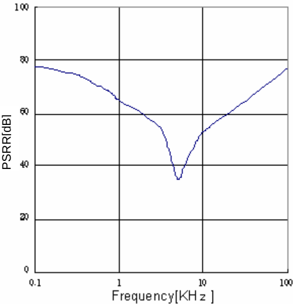
Figure 32. PSRR(Io=0mA)
