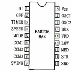
图 1 BA8206 BA4 的引脚说明
