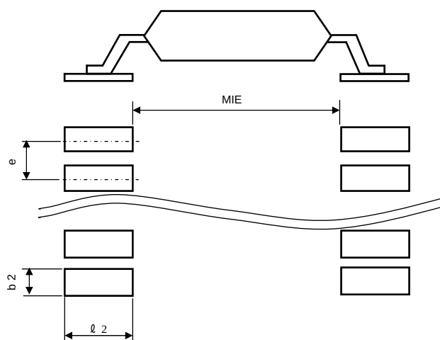
SOP8, SOP14, SSOP-B8 SSOP-B14, MSOP8
