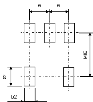
SSOP5
