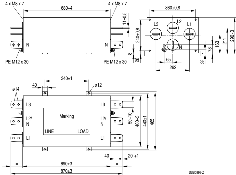
Maßbild B84144-G1600-S
