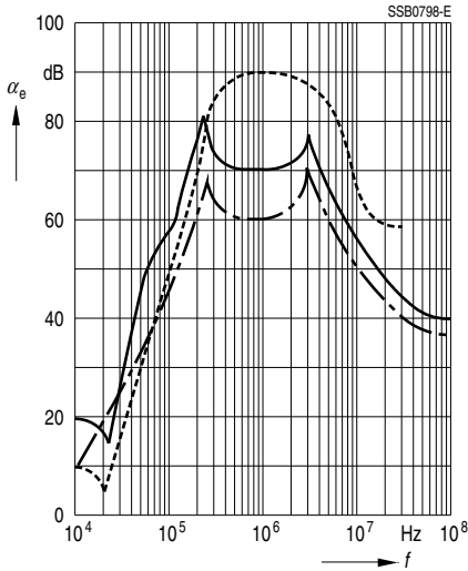
B84143-A16-R
