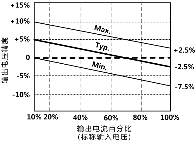
图 3. 输出电压 误差包络曲线图
