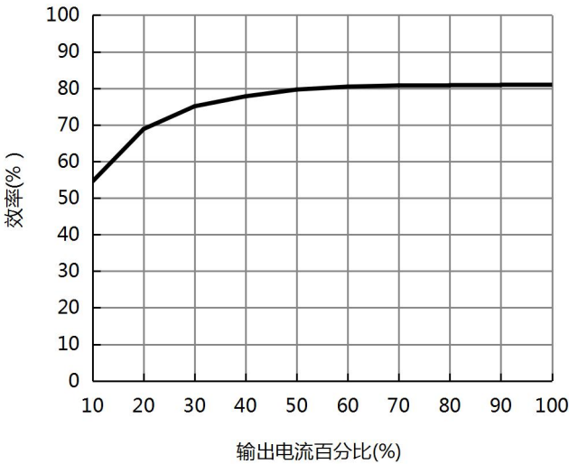
图 6. B0505LS-1W 效率 vs 输出负载 (标称输入)
