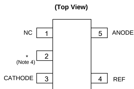
SOT25
