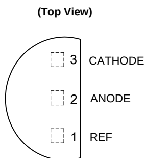
TO92 (Bulk Packing)
