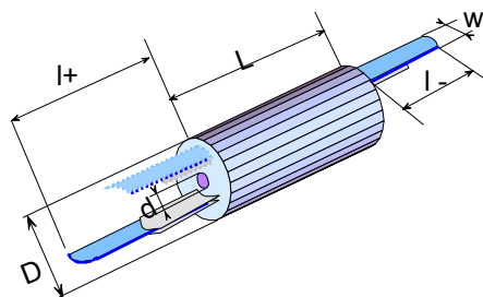
Dimensions
