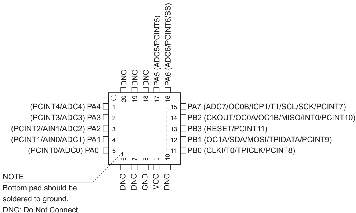
Figure 1-2. VQFN
