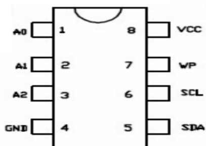
DIP8/SOP8/TSSOP8
