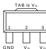
SOT-89 (Top View) APL5308
