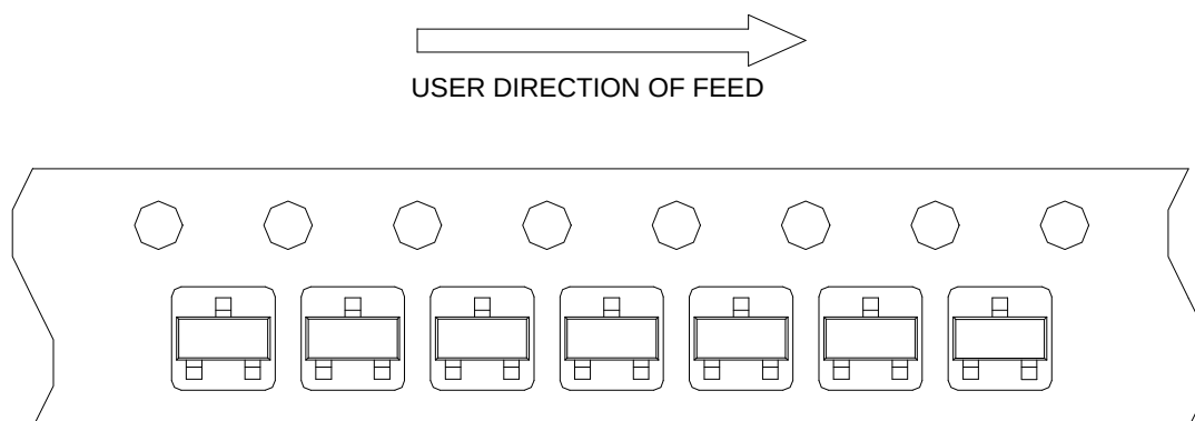
SOT-23-3
