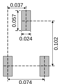
SOT-23
