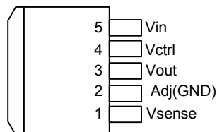
TO263-L
