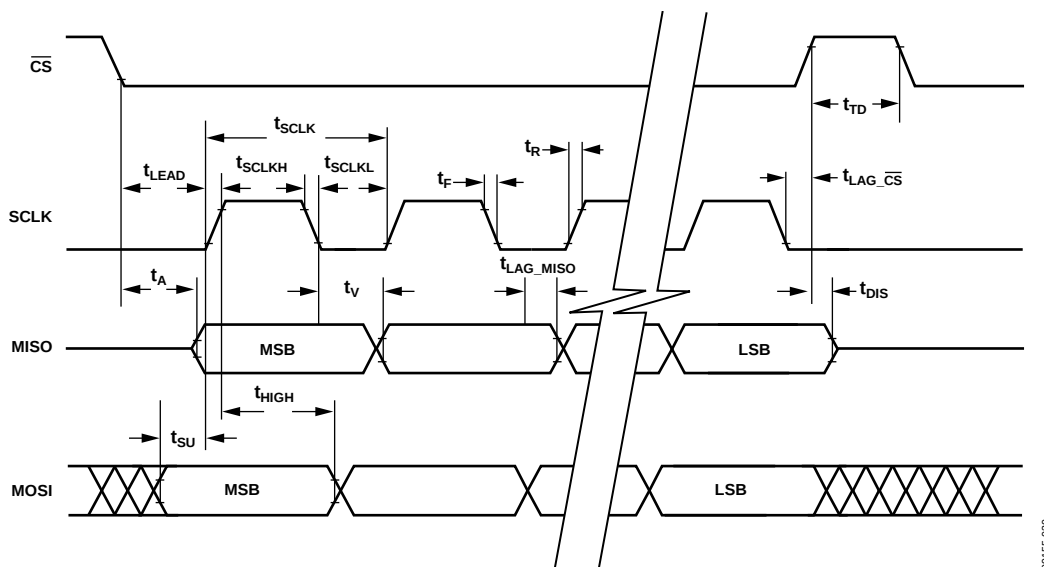
图31. SPI时序
