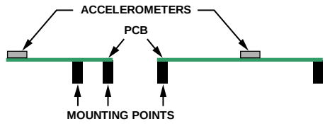
图45. 错误放置的加速度计
