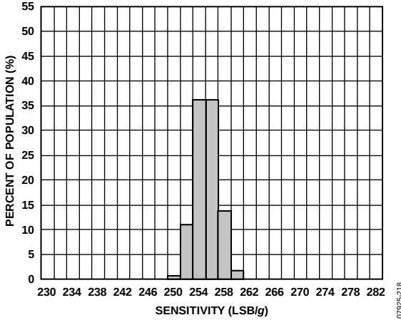
图18. 25 °C时的Z轴灵敏度, V_s = 2.5\text{ V} , 全分辨率
