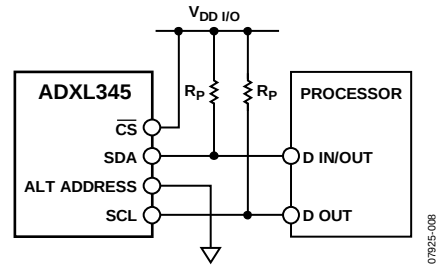
图40. I²C连接图(地址0x53)
