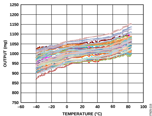
图15. Z轴1 g偏移与温度的关系—45个器件焊接到PCB, V_s = 2.5\text{ V}
