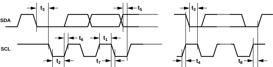
图3. I 2 C时序
