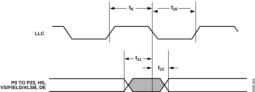
图4. 像素端口和控制SDR输出时序
