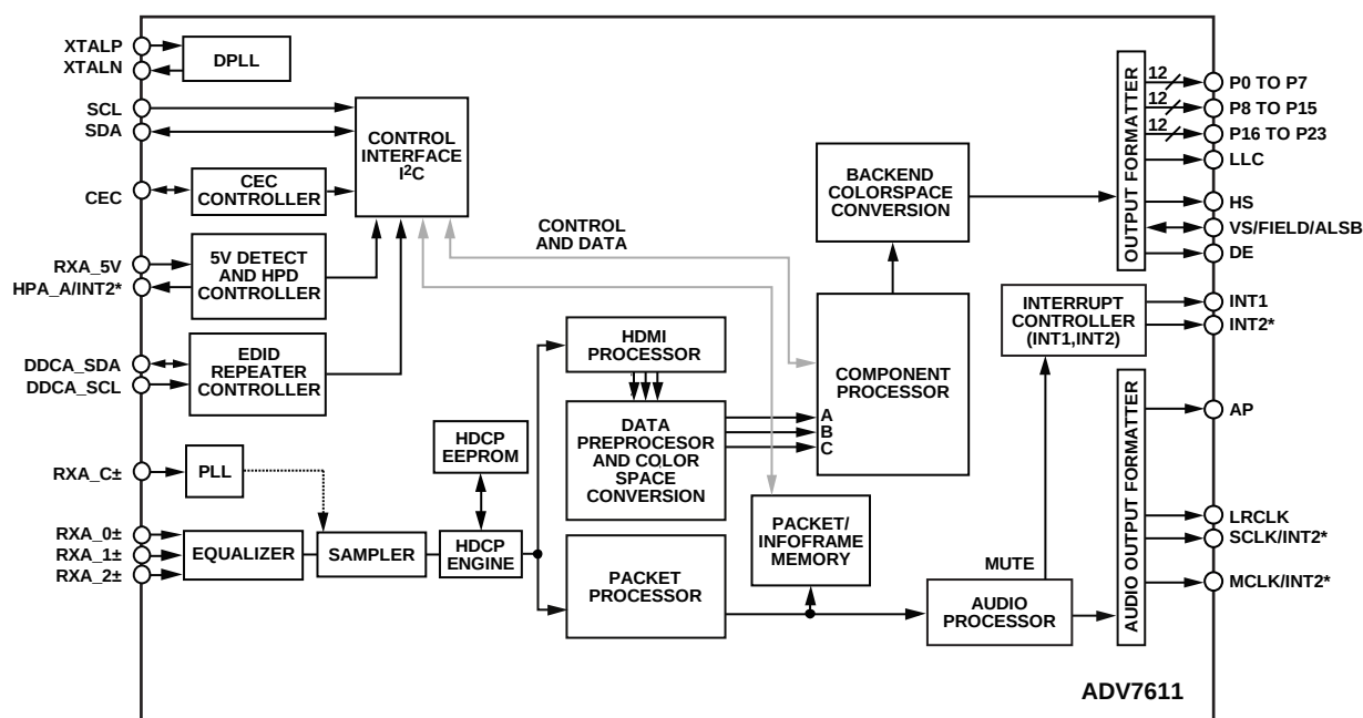
图2. 详细功能框图
