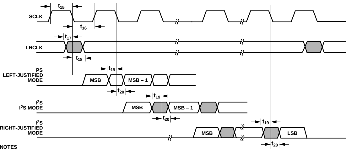
图5. I 2 S时序
