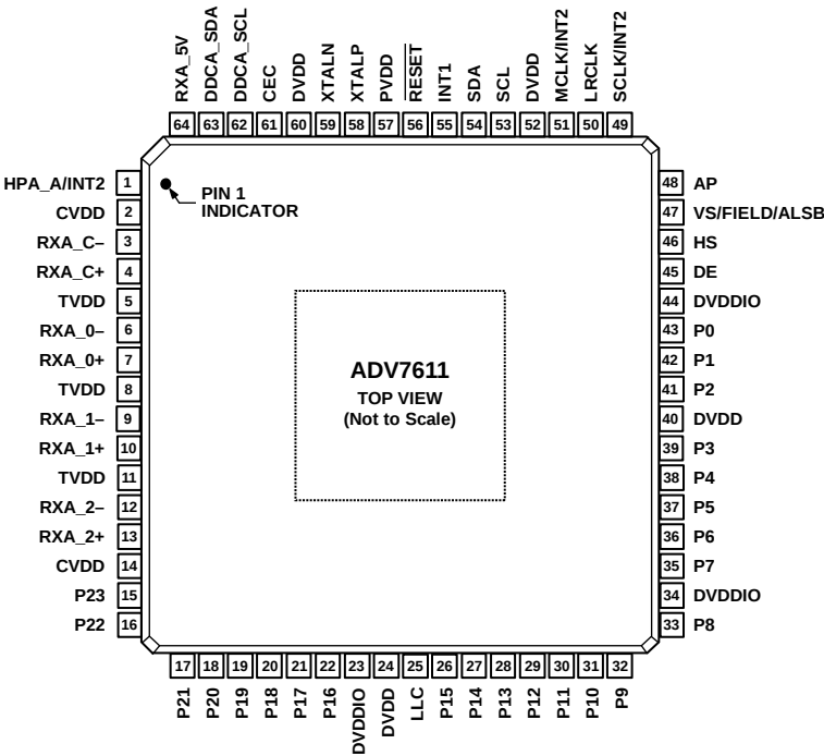
图6. 引脚配置
