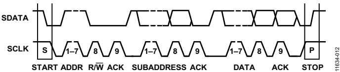
图12. 总线数据传输
