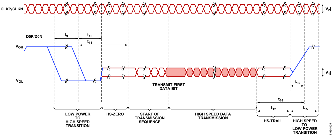
图3. ADV7280-M输出时序图(符合MIPI CSI-2规格)
