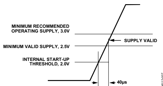
图7. 启动条件(电源压摆率 > 12.5 V/ms)
