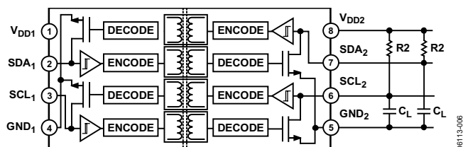
图6. ADuM1250框图
