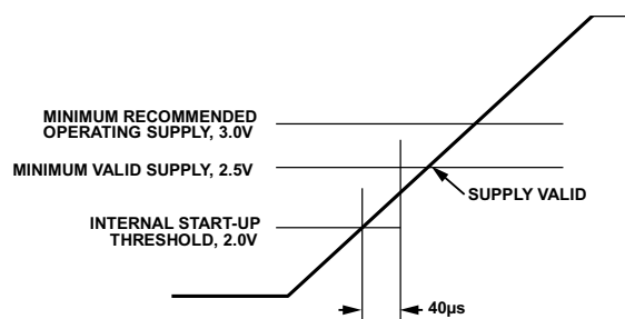
图8. 启动条件(电源压摆率 < 12.5 V/ms)
