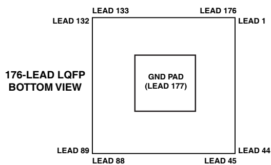
图73. 176引脚LQFP封装引脚配置 (底视图)
