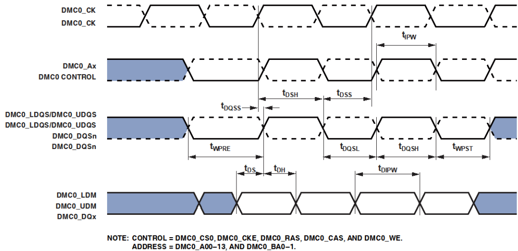
图13. DDR2 SDRAM控制器输出交流时序
