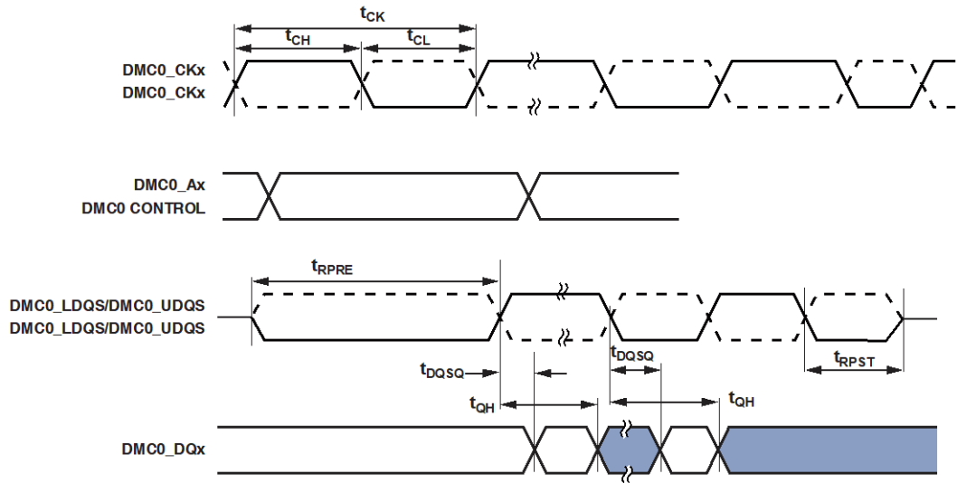
图12. DDR2 SDRAM控制器输入交流时序
