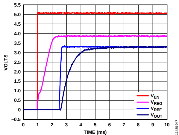
图47. V_{IN} 上升后的 V_{OUT} 、 V_{REF} 、 V_{REG} 启动时间, V_{OUT} = 3.3\text{ V} , V_{IN} = 5\text{ V}
