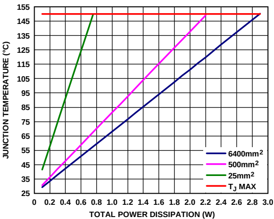
图61. 8引脚LFCSP的结温与总功耗的关系， T_A = 25^\circ\text{C}
