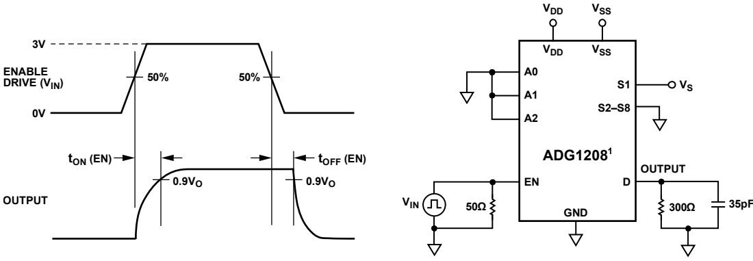
Figure 36. Enable Delay, t_{ON}(EN) , t_{OFF}(EN)
