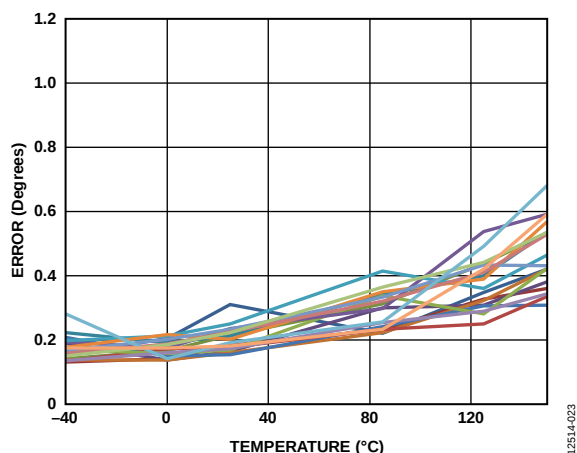
图16. 单点校准角度误差, V_{DD} = 2.7\text{ V} , GC = 关
