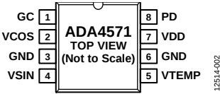
图2. 引脚配置
