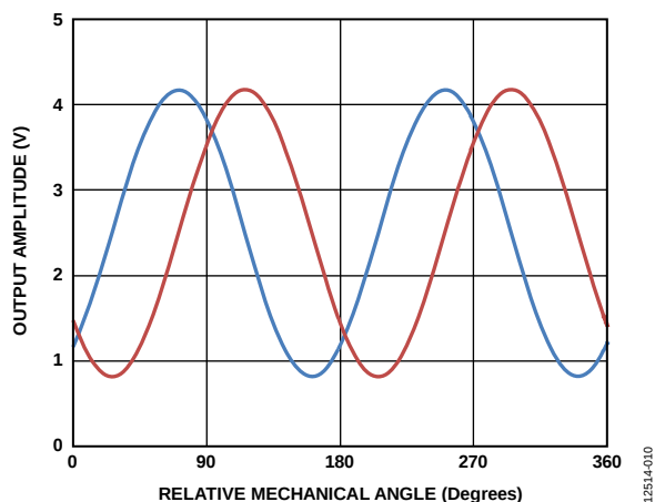
图3. 原始输出波形, V_{DD} = 5\text{ V} , GC = 开, T = 25^\circ\text{C}
