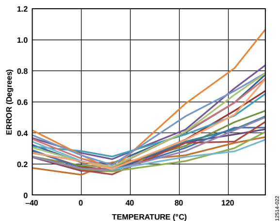
图15. 单点校准角度误差, V_{DD} = 2.7\text{ V} , GC = 开
