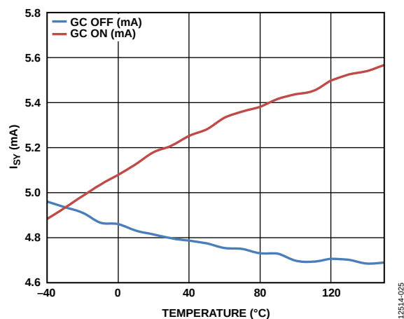
图18. 电源电流( I_{SY} )与温度的关系, V_{DD} = 5\text{ V}
