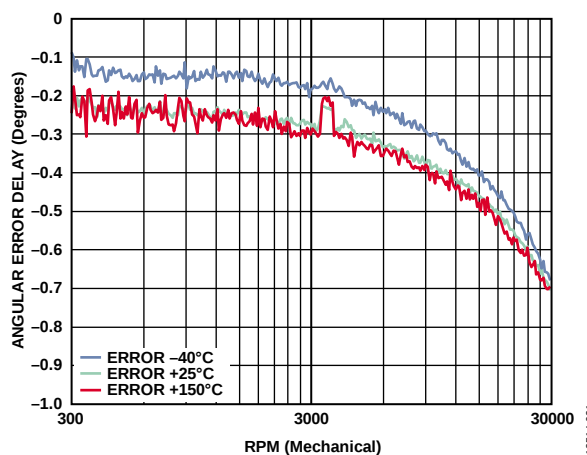
图24. 角度误差延迟与RPM(机械)的关系
