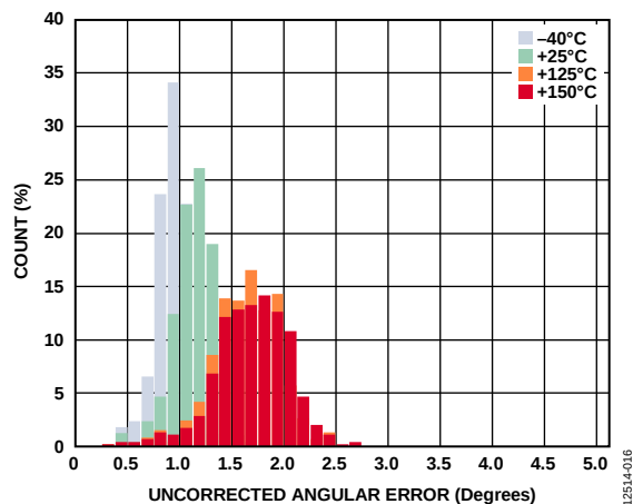
图9. 未校正角度误差, V_{DD} = 5.5\text{ V} , GC = 开
