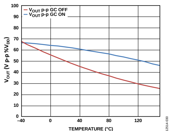
图23. 输出电压( V_{\text{SIN}} 和 V_{\text{COS}} )峰峰值与温度的关系(% V_{\text{DD}} )
