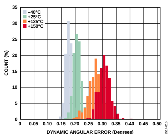
图8. 动态角度误差, V_{DD} = 2.7\text{ V} , GC = 关
