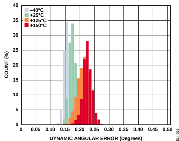
图6. 动态角度误差, V_{DD} = 5.5\text{ V} , GC = 关
