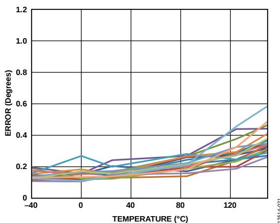
图14. 单点校准角度误差, V_{DD} = 5.5\text{ V} , GC = 关
