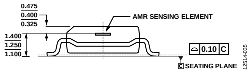
图31. ADA4571的断面图
