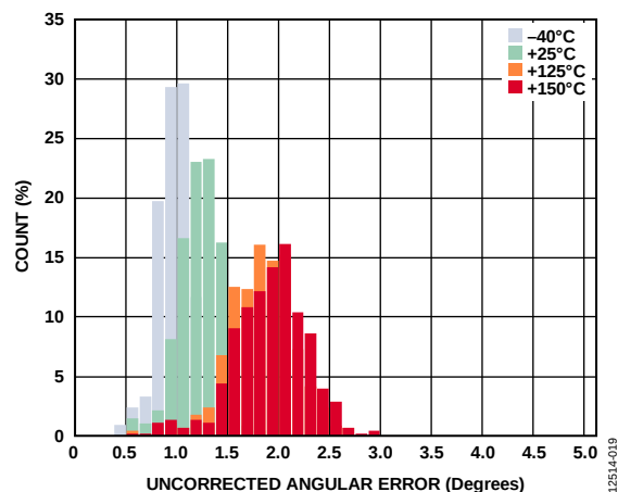
图12. 未校正角度误差, V_{DD} = 2.7\text{ V} , GC = 关
