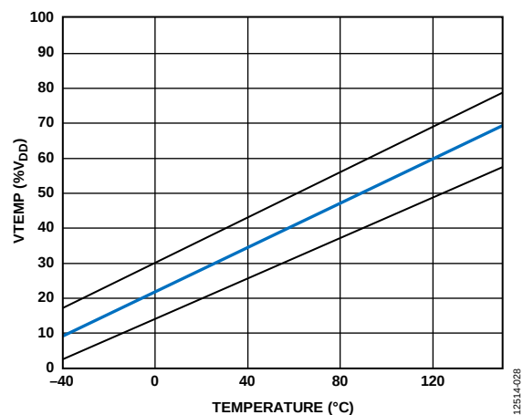
图21. VTEMP输出电压与温度的关系
