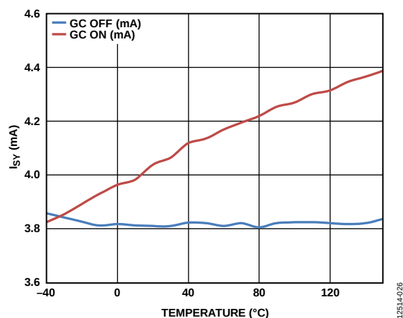
图19. 电源电流( I_{SY} )与温度的关系, V_{DD} = 3\text{ V}
