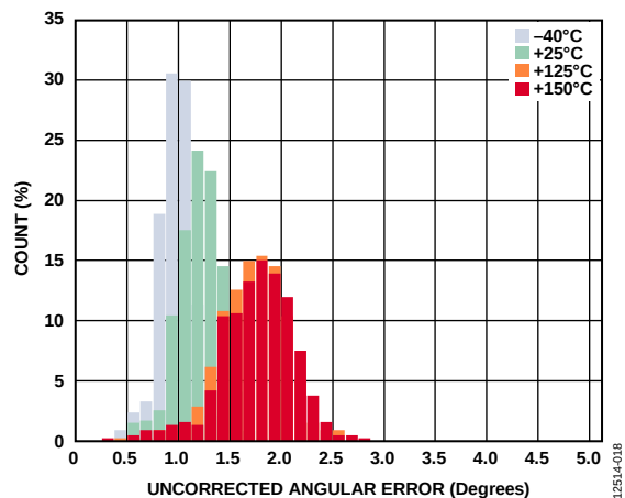
图11. 未校正角度误差, V_{DD} = 2.7\text{ V} , GC = 开
