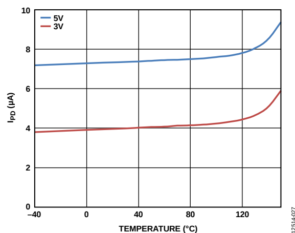
图20. 关断电流( I_{PD} )与温度的关系
