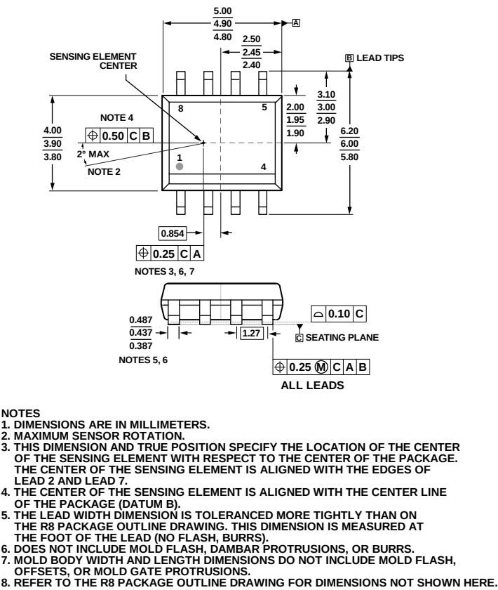
图30. ADA4571的机械图
