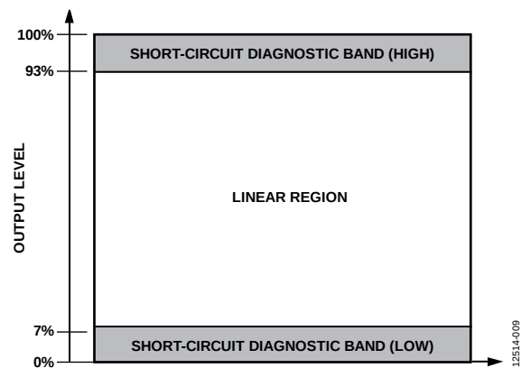
图34. 短路诊断状况中的输出范围分类
