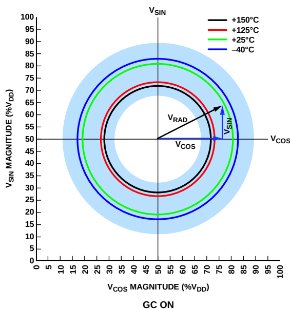
图32. GC开启时的半径值
