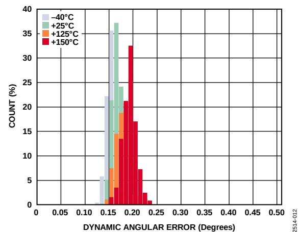
图5. 动态角度误差, V_{DD} = 5.5\text{ V} , GC = 开
