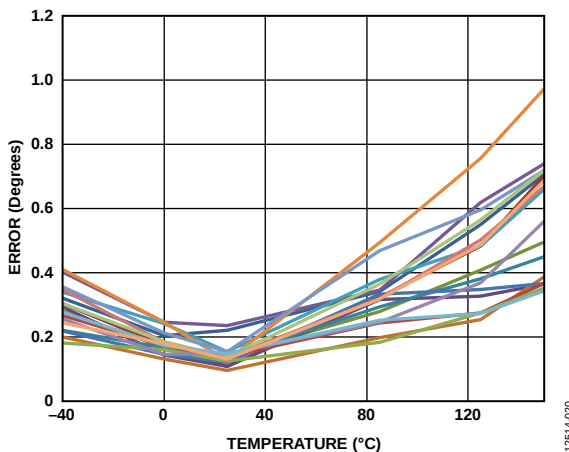
图13. 单点校准角度误差, V_{DD} = 5.5\text{ V} , GC = 开
