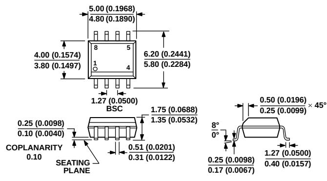
图35. 8引脚标准小型封装[SOIC_N] 窄体 (R-8) 图示尺寸单位：mm和(inch)
