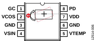
图25. 绑定排列和封装中的传感器对齐
