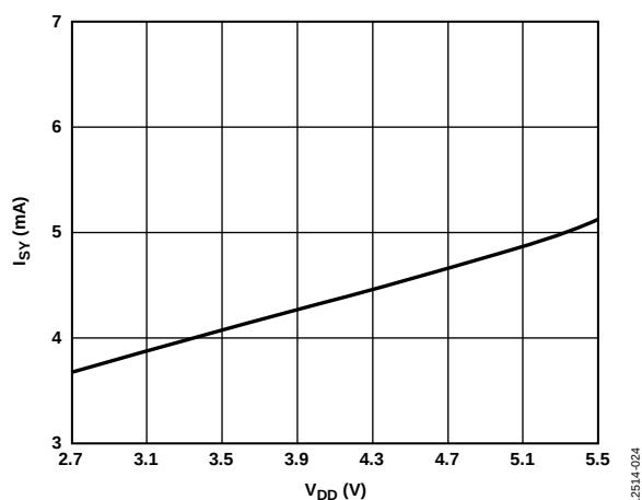
图17. 电源电流( I_{SY} )与电压( V_{DD} )的关系, T = 25\text{ °C}
