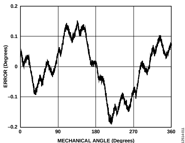
图4. 失调校正后的误差波形, V_{DD} = 5\text{ V} , GC = 开
