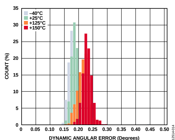
图7. 动态角度误差, V_{DD} = 2.7\text{ V} , GC = 开
