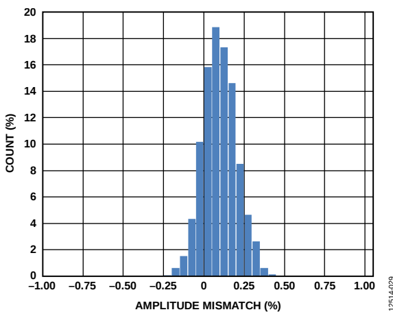
图22. 幅度同步(% k)
