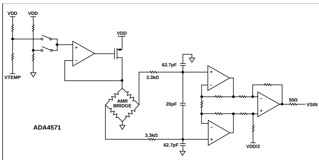
图27. ADA4571正弦通道内部详细框图
