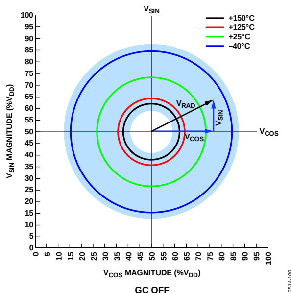
图33. GC关闭时的半径值
