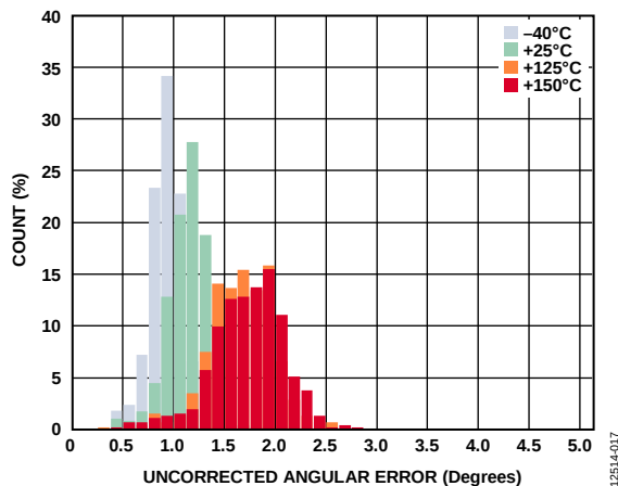
图10. 未校正角度误差, V_{DD} = 5.5\text{ V} , GC = 关
