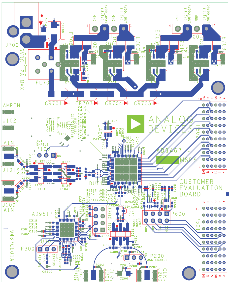
Figure 24. Top (Layer 1)
