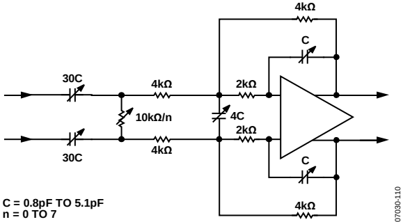
图54. 滤波器原理示意图
