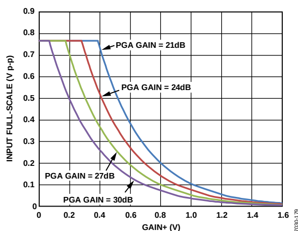
图50. LNA(21.3 dB增益设置)/VGA满量程范围
