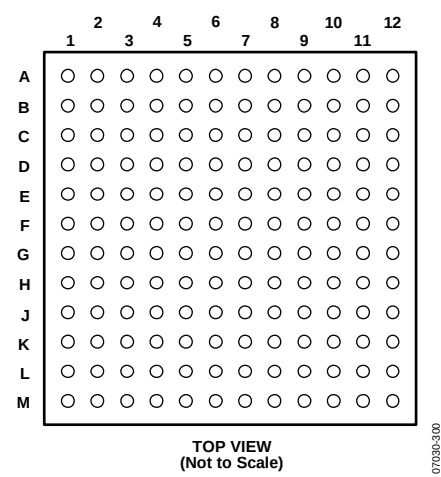
图5. BGA引脚配置
