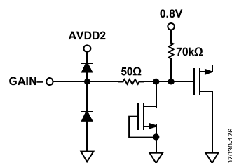
图35. 等效GAIN-输入电路
