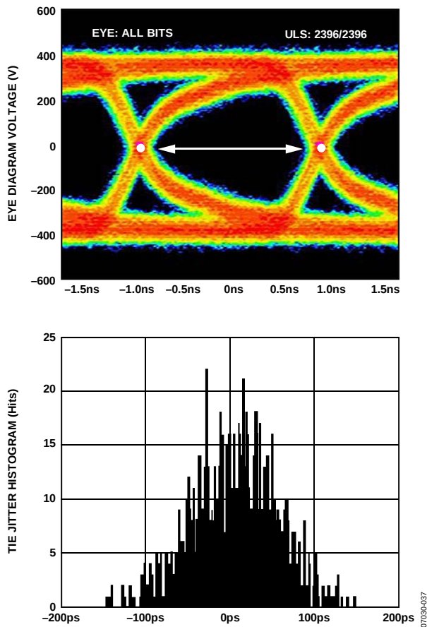
图67. LVDS输出的数据眼(ANSI-644模式, 100 \Omega 端接电阻, 走线长度大于24英寸, 标准FR-4)
