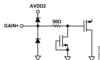
图34. 等效GAIN+输入电路
