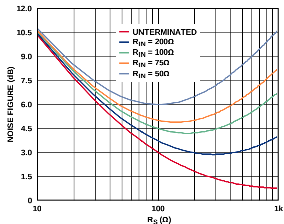
图43. 各种 R_{IN} 固定值, 有源端接匹配输入, V_{GAIN} = 0.8 \text{ V} 时噪声系数和 R_S 的关系
