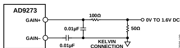
图52. 单端GAIN±引脚配置
