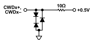
图36. 等效CWDx±输出电路
