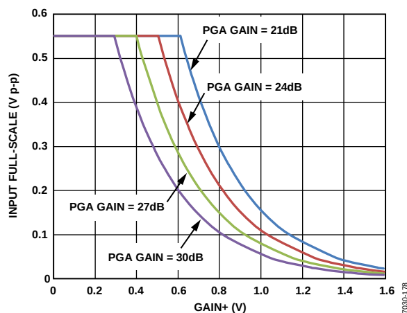
图49. LNA(17.9 dB增益设置)/VGA满量程范围
