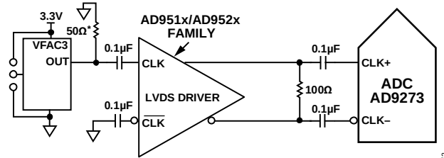
图57. 差分LVDS采样时钟
