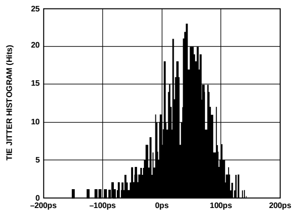
图65. LVDS输出的数据眼(ANSI-644模式, 走线长度小于24英寸, 标准FR-4)
