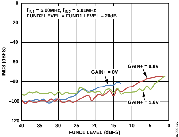
图24. IMD3与基波幅度(FUND1)电平的关系
