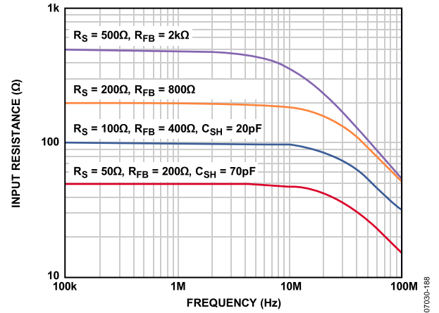
图40. 各种 R_{FB} 值时 R_{IN} 与频率的关系 (同时显示 R_S 和 C_{SH} 的影响)
