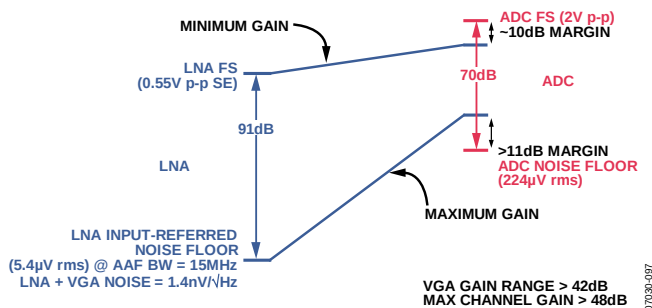
图47. 12位40 MSPS ADC的TGC运行增益要求
