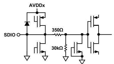
图28. 等效SDIO输入电路
