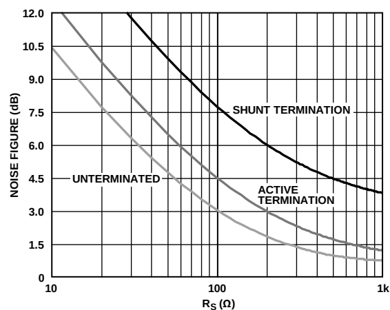
图42. 分流器端接、有源端接匹配和无端接输入时的噪声系数和 R_S 的关系, V_{GAIN} = 0.8 \text{ V}
