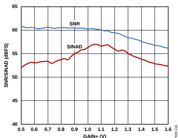
图16.信噪比/信噪失真比与 GAIN+ 的关系, A_{IN} = -1.0\text{ dBFS}
