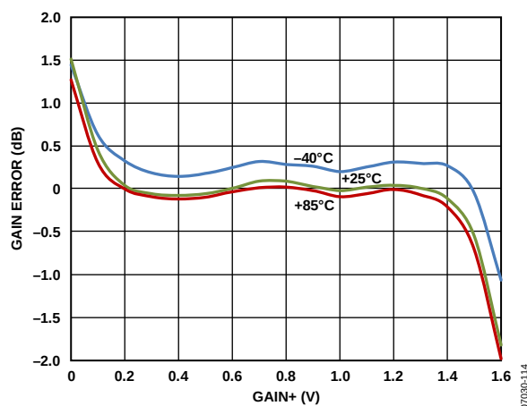
图6. 三种温度下增益误差与GAIN+的关系
