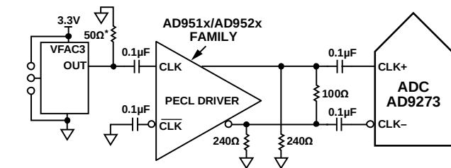
图56. 差分PECL采样时钟
