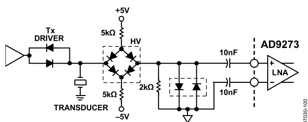
图44. 输入过载保护
