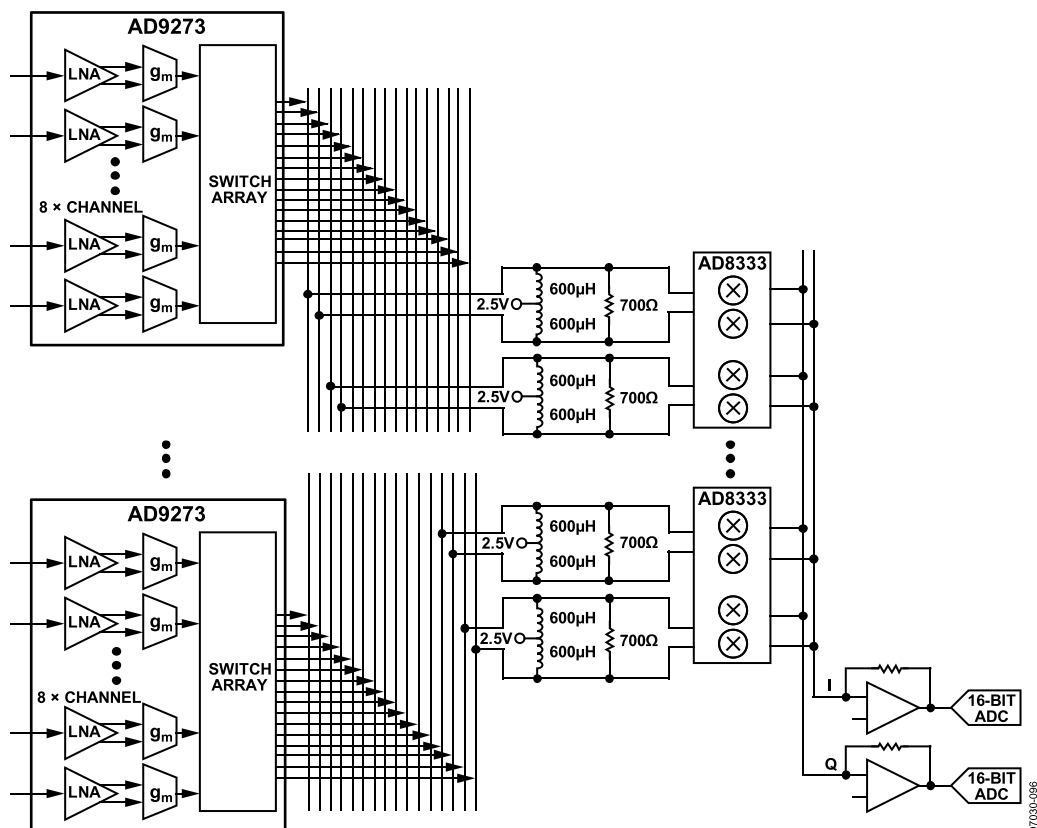
图45. 使用CWDx±输出的AD8333或AD8339典型连接接口
