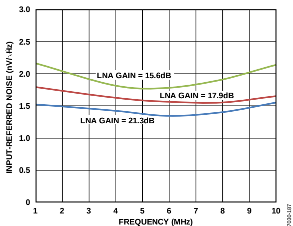
图14. 短路, 折合到输入的噪声与频率的关系, PGA 增益 = 30\text{ dB} , GAIN+ = 1.6\text{ V}
