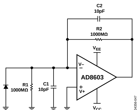
图47. 光电二极管电路
