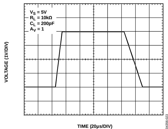
图23. 大信号瞬变
