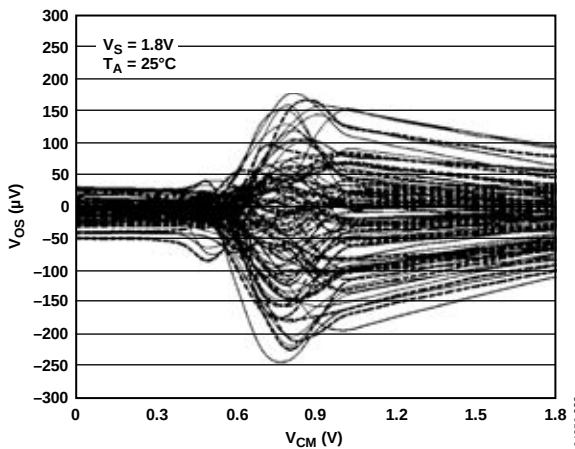
图29. 输入失调电压与共模电压的关系
