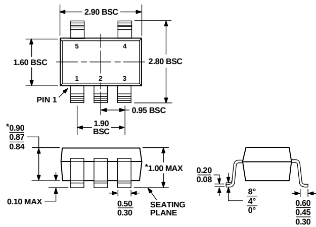
图48. 5引脚超薄小型晶体管封装[TSOT] (UJ-5) 图示尺寸单位: mm
