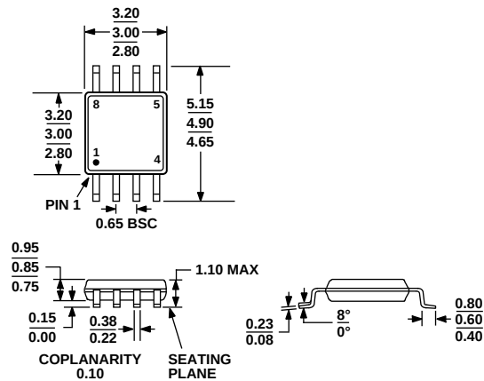
图49. 8引脚超小型MSOP封装 (RM-8) 图示尺寸单位: mm
