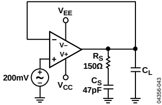
图43.缓冲器网络
