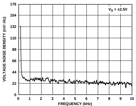
图27. 电压噪声密度与频率的关系
