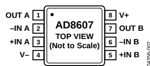
图2. 8引脚MSOP(RM后缀)
