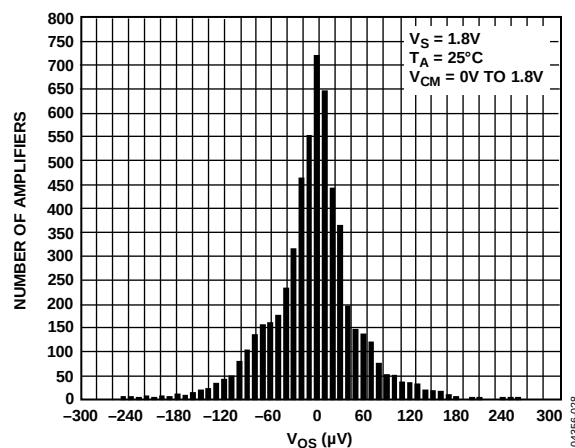
图28. V_{OS} 分布
