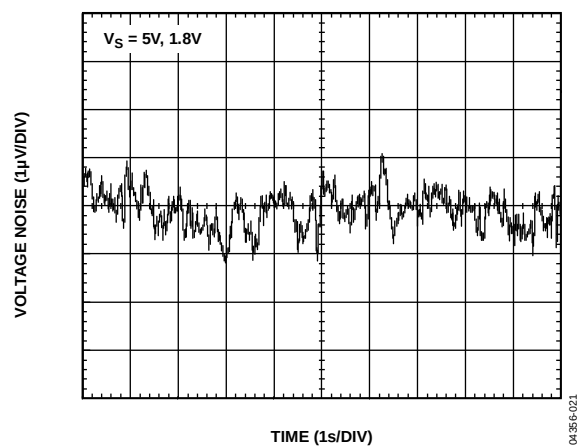
图21. 0.1 Hz至10 Hz输入电压噪声
