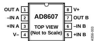
图3. 8引脚SOIC(R后缀)
