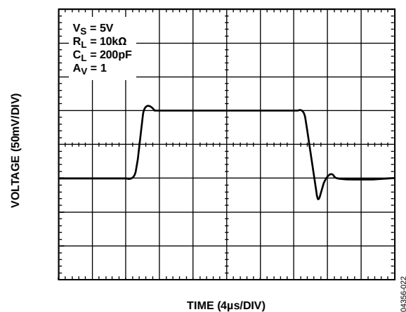
图22. 小信号瞬变
