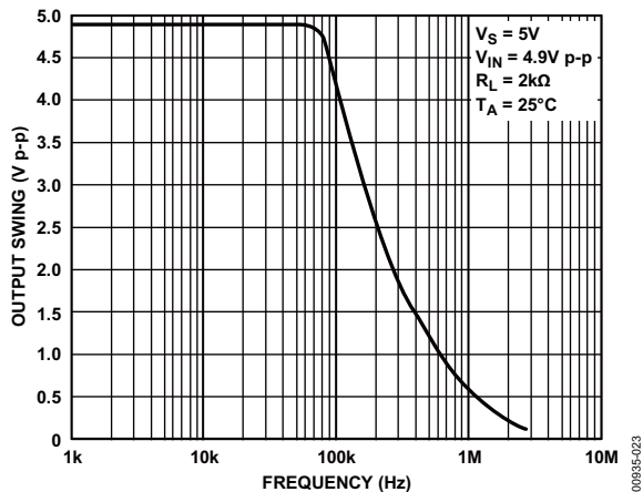
图24. 闭环输出电压摆幅与频率的关系
