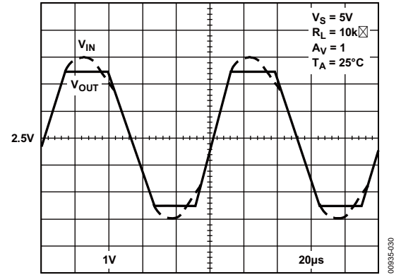
图31. 无倒相
