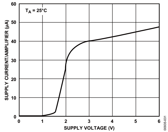
图32. 每个放大器的电源电流与电源电压的关系
