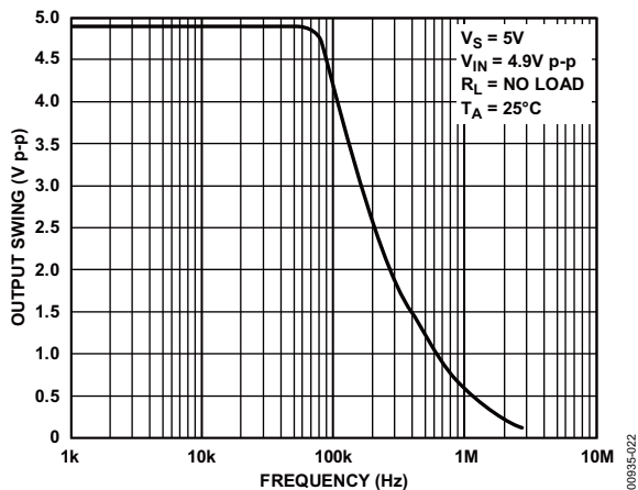
图23. 闭环输出电压摆幅与频率的关系
