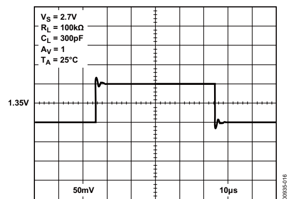
图16. 小信号瞬态响应
