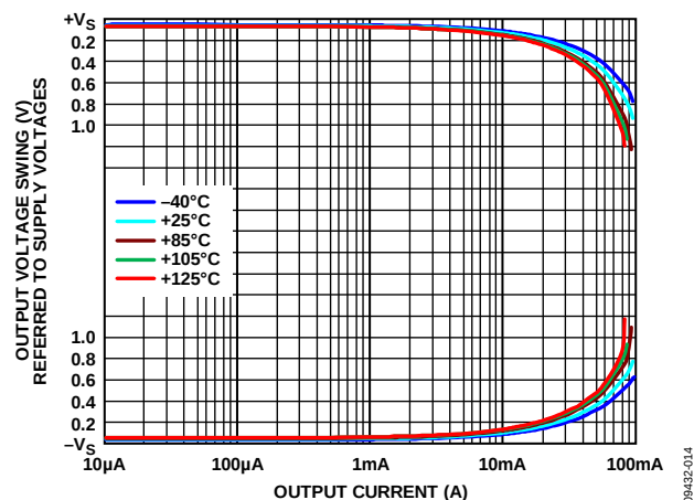
图14. 输出电压摆幅与输出电流及温度的关系, V_S = \pm 5\text{ V} 和 +5\text{ V}
