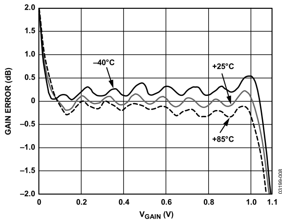
图8. 三种温度下绝对增益误差与 V_{\text{GAIN}} 的关系
