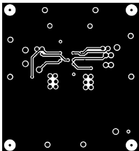
图108. 原边铜结构
