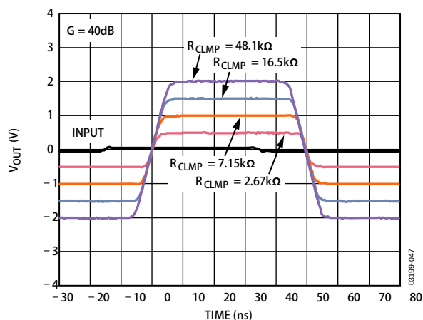
图47. 四个值 R_{\text{CLMP}} 下的箝位电平脉冲响应
