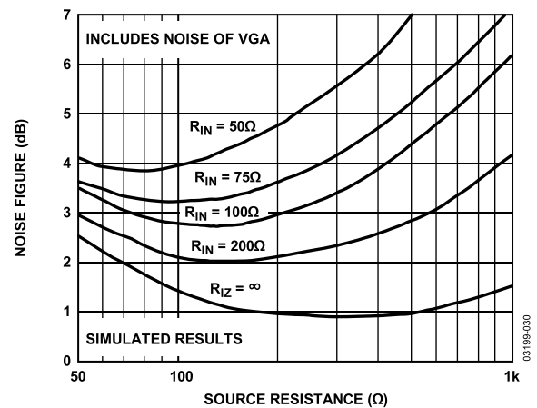
图30. 不同 R_{IN} 值下的噪声系数与 R_S 的关系
