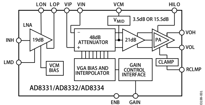
图1. 信号路径功能框图
