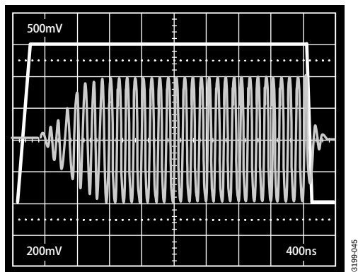
图45. 引脚 G_{\text{AIN}} 瞬变响应, 顶部: V_{\text{GAIN}} , 底部: 输出电压
