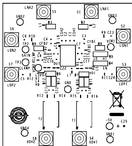
图107. AD8332-EVALZ装配图
