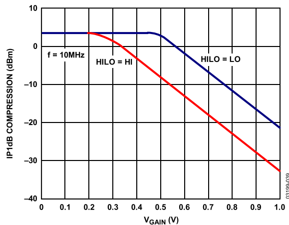
图39. IP1dB压缩与 V_{GAIN} 的关系
