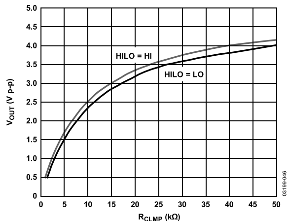
图46. 箝位电平与 R_{\text{CLMP}} 的关系
