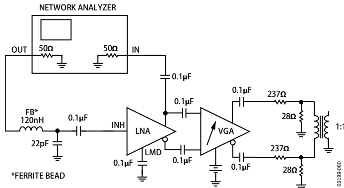
图60. 测试电路—频率响应(末端接LNA，单端)
