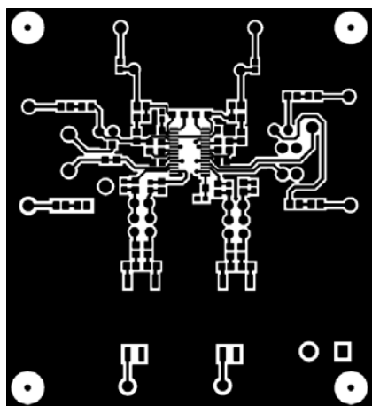
图108. 原边铜结构
