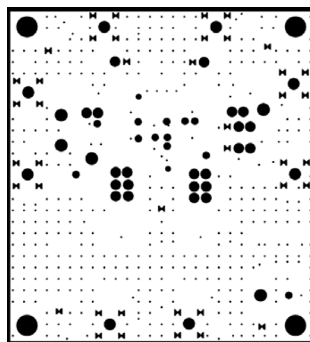
图110. 接地层
