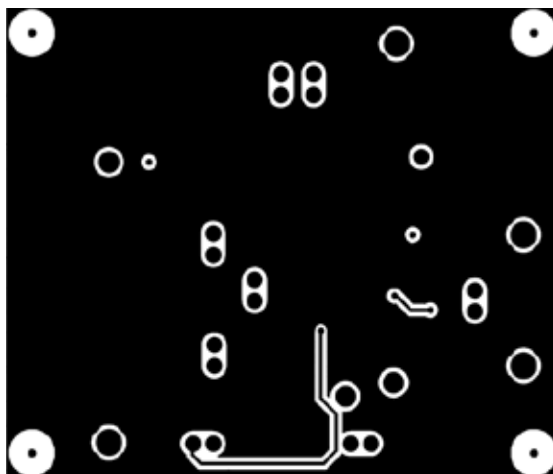
图100. 副边铜结构
