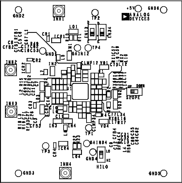
图114. AD8334-EVALZ装配图
