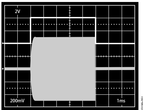
图50. VGA过驱恢复, V_{INH} 4 mV p-p至275 mV p-p突发, 显示 V_{GAIN} = 1 V VGA输出, 衰减24 dB
