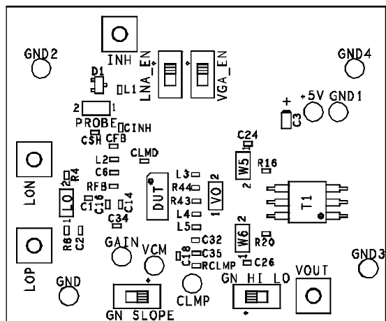
图98. AD8331-EVALZ装配图
