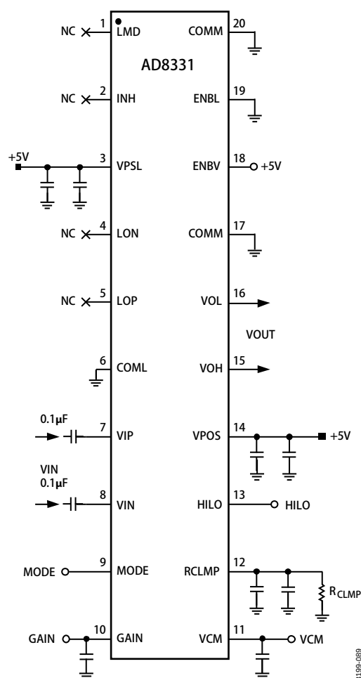
图90. 禁用LNA
