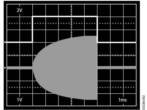
图52. 使能响应, 大信号, 顶部: V_{ENB} , 底部: V_{OUT} , V_{INH} = 150 mV p-p
