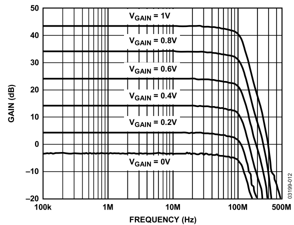
图12. 不同 V_{\text{GAIN}} 值下的频率响应
