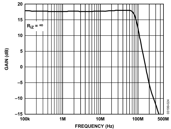
图24. 频率响应(末端接LNA, 单端)
