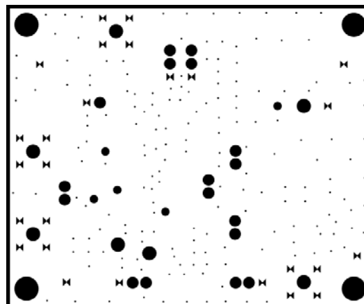
图101. 内层接地
