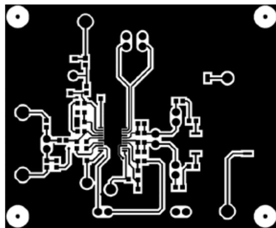
图99. 原边铜结构
