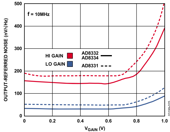
图25. 折合到输出端的噪声与 V_{GAIN} 的关系
