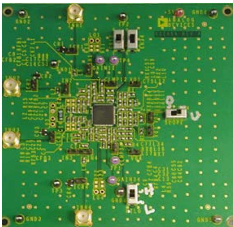
图113. AD8334-EVALZ俯视图
