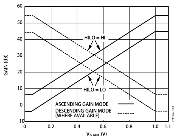
图73. 理想增益控制特性
