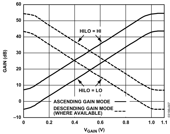
图7. 增益与 V_{\text{GAIN}} 和MODE的关系(RU封装提供MODE)
