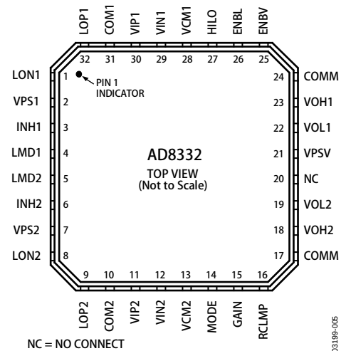
图5. 32引脚LFCSP引脚配置(AD8332)
