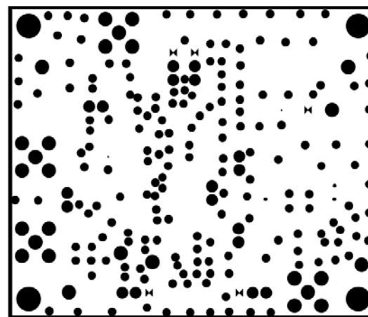
图102. 电源层
