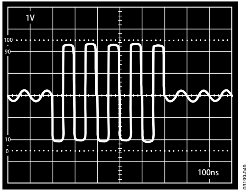
图49. VGA过驱恢复, V_{INH} 4 mV p-p至70 mV p-p突发, 显示 V_{GAIN} = 1 V VGA输出, 衰减24 dB
