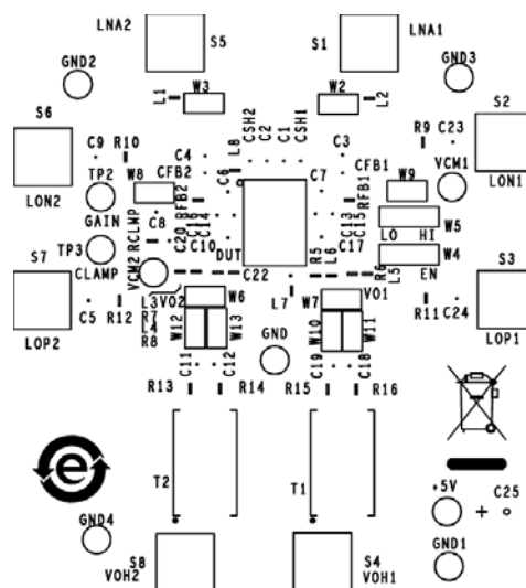
图112. 器件侧丝网图
