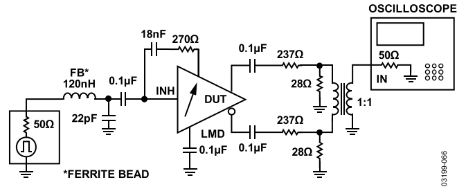
图66. 测试电路—脉冲响应测量
