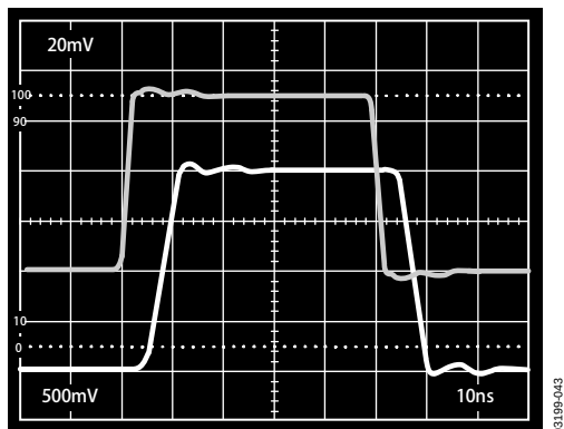
图43. 大信号脉冲响应, G = 30 \text{ dB} , \text{HILO} = \text{HI} 或 \text{LO} , 顶部: 输入电压, 底部: 输出电压
