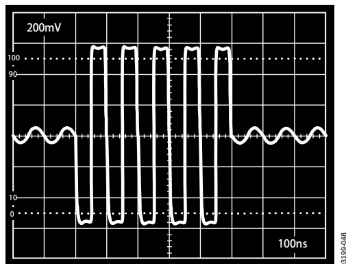
图48. LNA过驱恢复, V_{\text{INH}} 0.05 \text{ V p-p} 至 1 \text{ V p-p} 突发, 显示 V_{\text{GAIN}} = 0.27 \text{ V VGA} 输出
