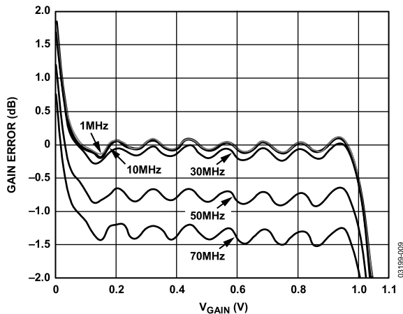
图9. 不同频率下绝对增益误差与 V_{\text{GAIN}} 的关系
