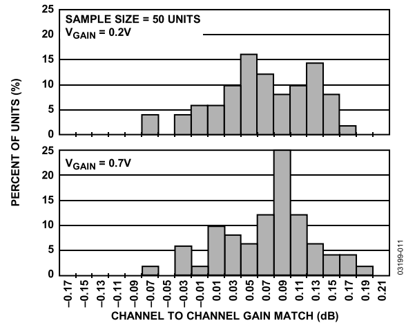
图11. 增益匹配直方图( V_{\text{GAIN}} = 0.2\text{ V} 和 0.7\text{ V} )
