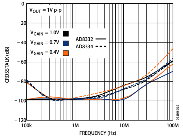
图16. 不同 V_{\text{GAIN}} 值下的通道间串扰与频率的关系
