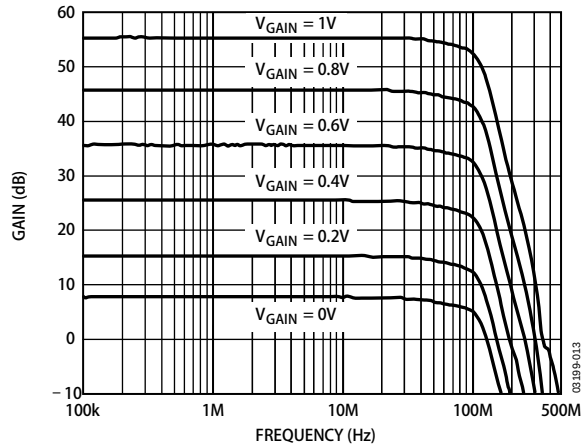
图13. 不同 V_{\text{GAIN}} 值下的频率响应(HILO = HI)
