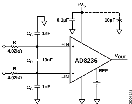
图40. 射频干扰(RFI)抑制
