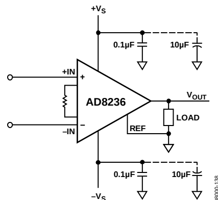
图37. 电源去耦、REF及以接地为基准的输出
