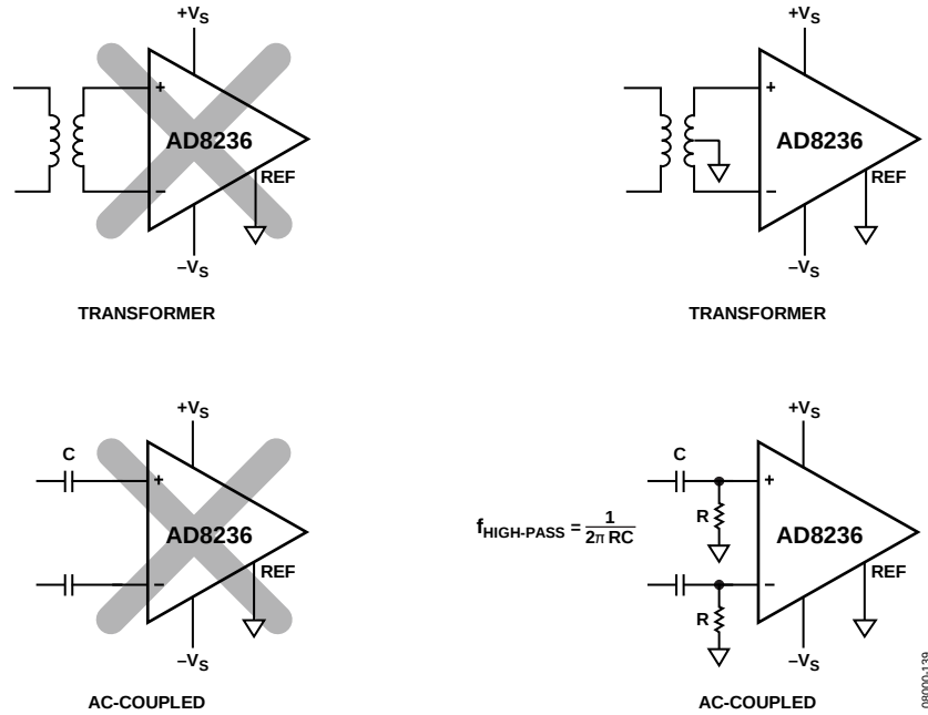
图38. 创建一条 I_{BIAS} 返回路径
