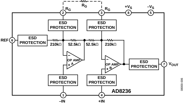
图34. 简化原理图
