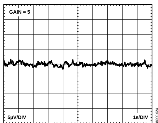
图8. 0.1 Hz至10 Hz折合成到输入端电压噪声
