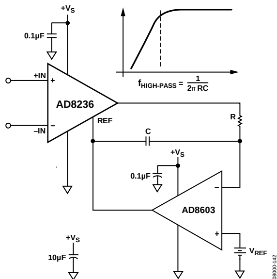
图41. 交流耦合电路
