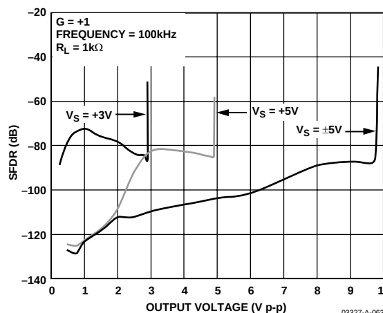
图2 SFDR与输出幅度的关系
