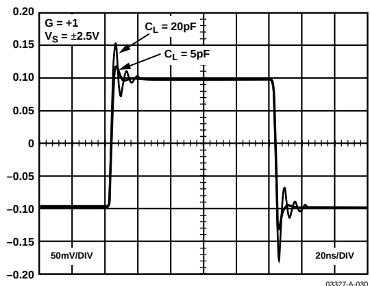
图31. 容性负载下的小信号瞬态响应
