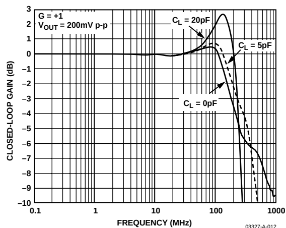
图13. 不同 C_{LOAD} 下的AD8028小信号频率响应
