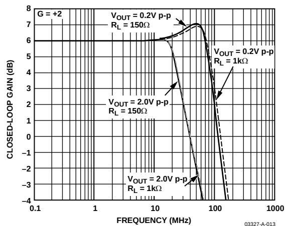
图14. 不同 R_{LOAD} 值下的小信号频率响应
