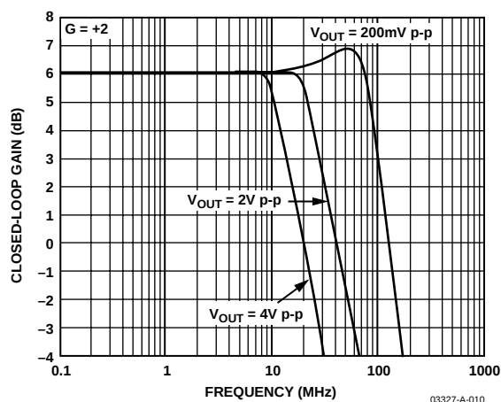
图11. 不同输出幅度下的频率响应
