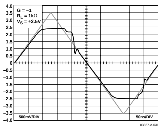
图32. 输出过驱恢复
