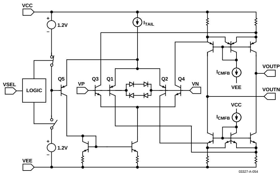
图55. 简化输入级
