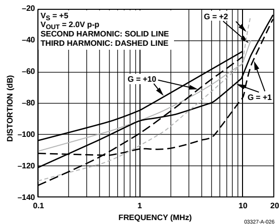
图27. 谐波失真与频率和增益的关系
