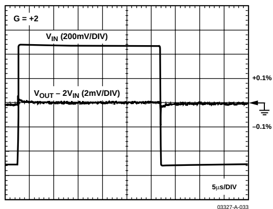
图34. 长期建立时间
