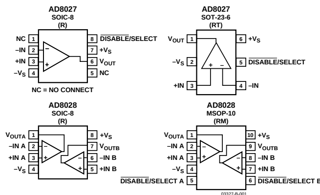
图1 连接图(顶视图)
