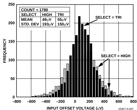
图38. 输入失调电压分布图
