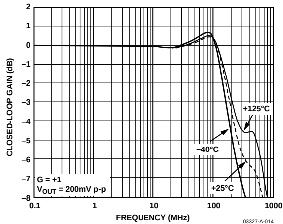
图15. AD8028小信号频率响应与温度的关系
