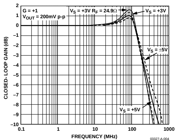
图5. 不同电源下的AD8027小信号频率响应
