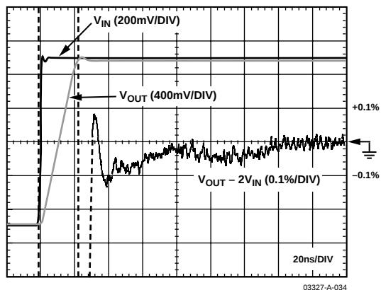
图35. 0.1%短期建立时间
