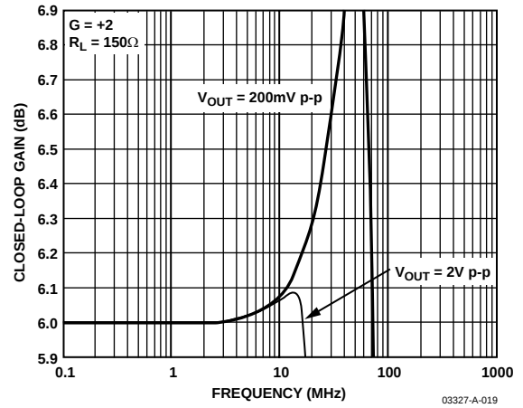
图20. 0.1 dB平坦度频率响应
