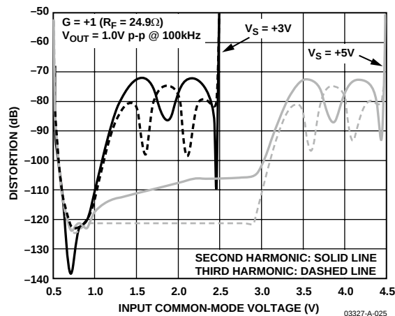
图26. 谐波失真与输入共模电压的关系, SELECT = 三态或开路
