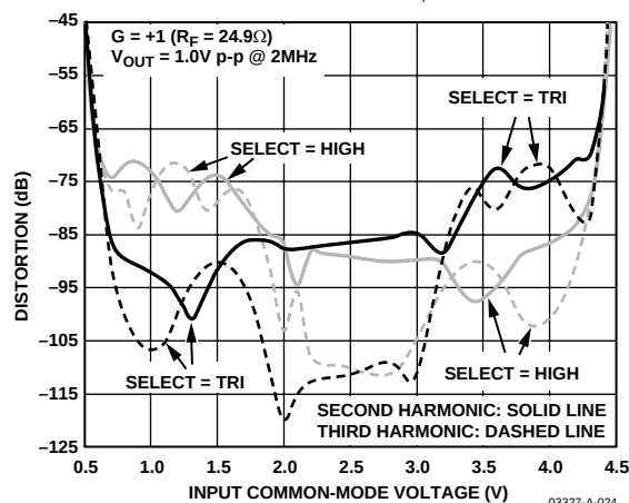
图25. 谐波失真与输入共模电压的关系, V_S = 5V
