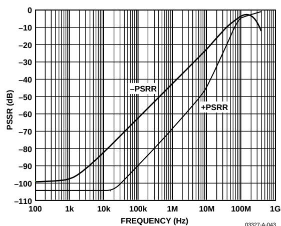
图44. PSRR与频率的关系
