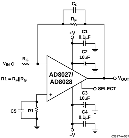
图58. 宽带反相增益配置
