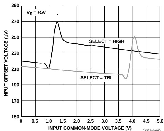
图41. 输入失调电压与输入共模电压的关系, V_S = 5
