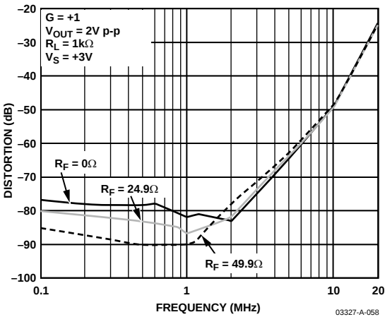
图59. SFDR与频率和不同R F 的关系
