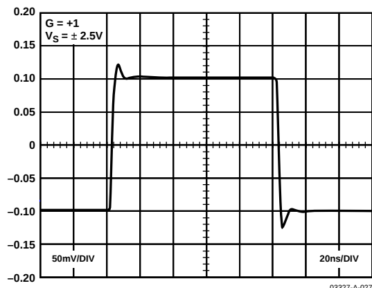
图28. 小信号瞬态响应
