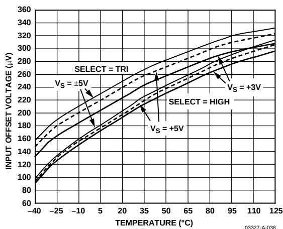
图39. 输入失调电压与温度的关系
