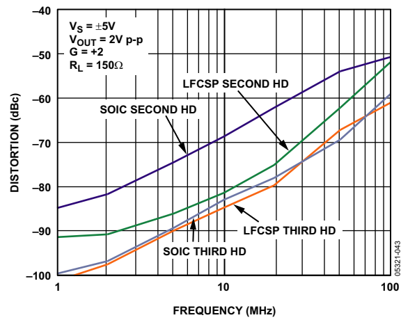
图22. 谐波失真与频率的关系
