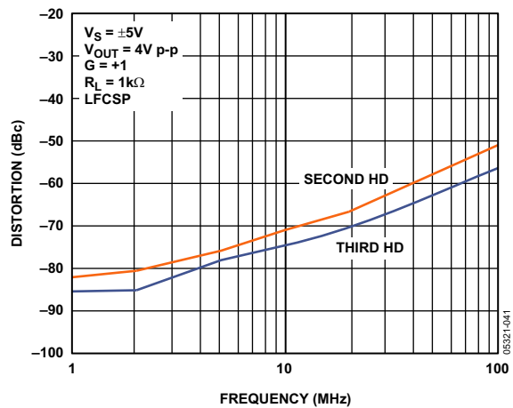
图21. 谐波失真与频率的关系
