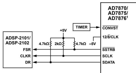
Figure 29. ADSP-2101/ADSP-2102 Serial Interface
